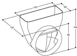
A: ø 152.5
