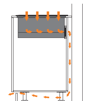
Ungeführte Umluft Set CA082011
