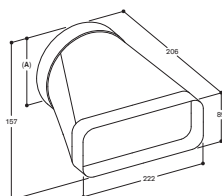
A: ø 152.5
