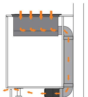
Geführte Umluft Set CA082061
