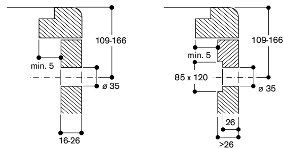
Werkbladafzuiging VL 410
