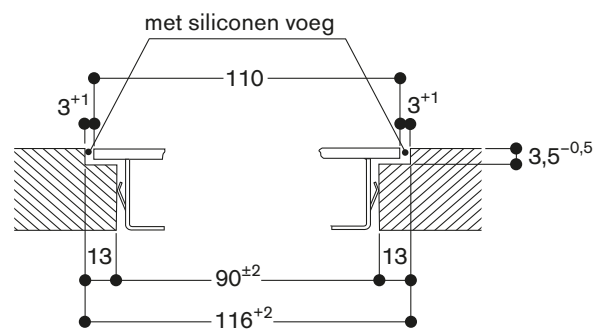
Doorsnede in de lengte
