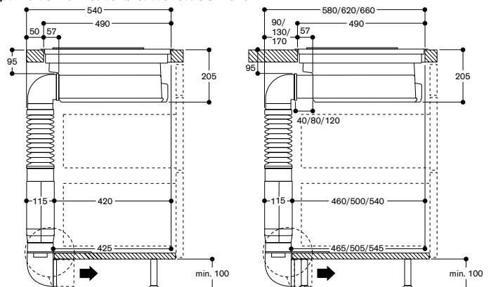
Zijaanzicht CV 282 met luchtcirculatiemodule CA 282 811
