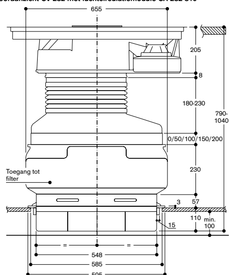
Vooraanzicht CV 282 met luchtcirculatiemodule CA 282 810
