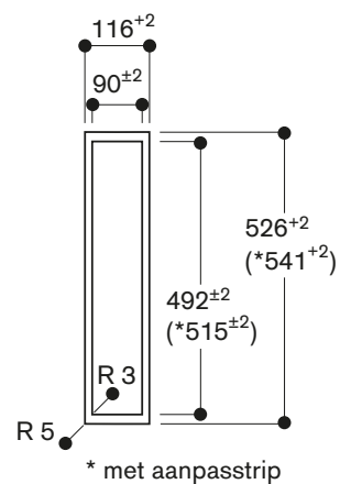
Aanzicht van boven
