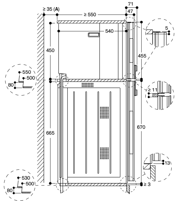
Zijaanzicht BS 484/485 boven BO
