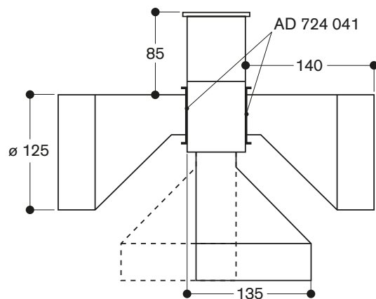
VL 414 met AD 724 041
