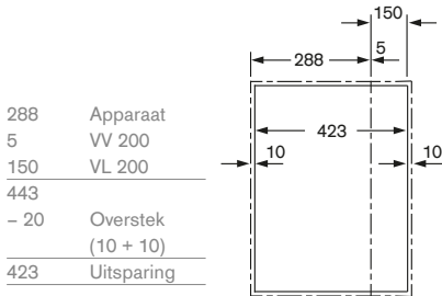
Uitsparingsformaten voor de Vario 200 serie in combinatie met werkbladafzuiging.
