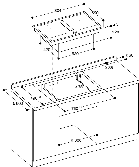
Afmeting in mm
