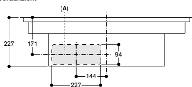
A: Direct op de achterzijde aangesloten
