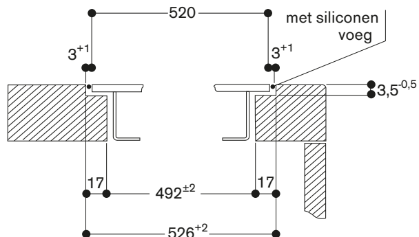
Dwarsdoorsnede
