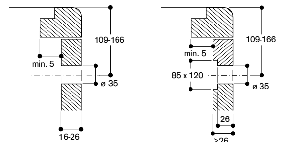
Werkbladafzuiging VL 410
