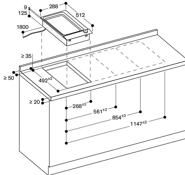
Afmeting in mm
