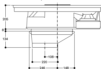
Vooraanzicht CV 282 met platte buis-aansluitstuk CA 284 010
