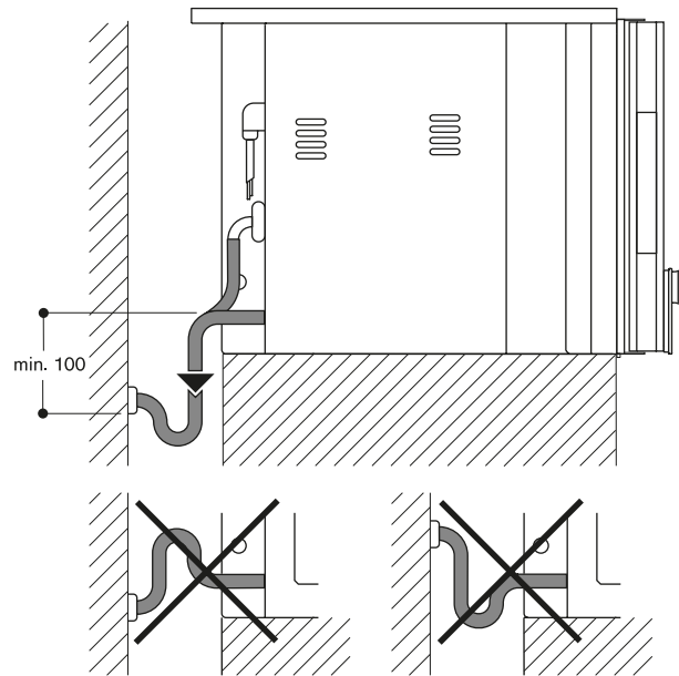
Waterafvoer-aansluiting
