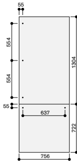
Nisbreedte 76,2 cm
