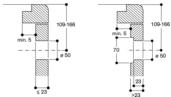
Inductiekookzones CI 422
