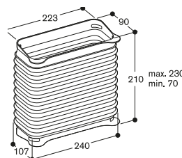
AD 410 040: Flexibel aansluitstuk voor de VL 200, DN 150 vlak.
