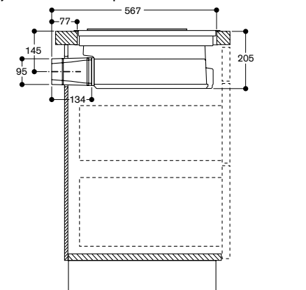
Zijaanzicht CV 282 met platte buis-aansluitstuk CA 284 010
