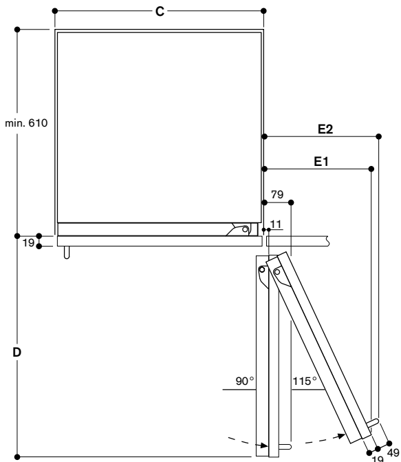
Wandafstand RB 472/RC/RF/RW
