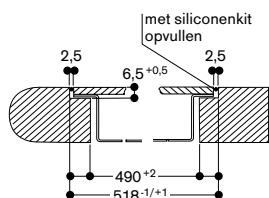
Dwarsdoorsnede
