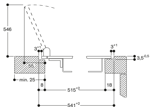
Installatie met deksel; Vlakke inbouw.
