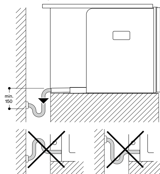
Afvalwateraansluiting
