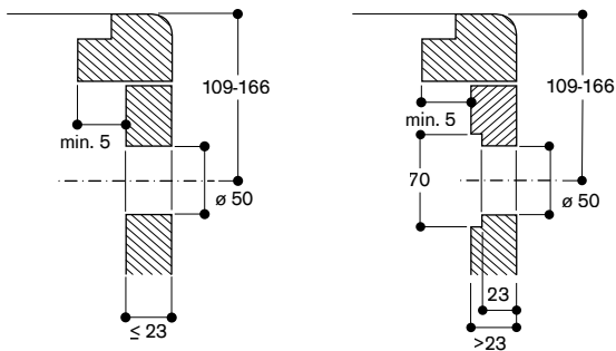
Inductiekookzones CI 414 &amp; CI 422
