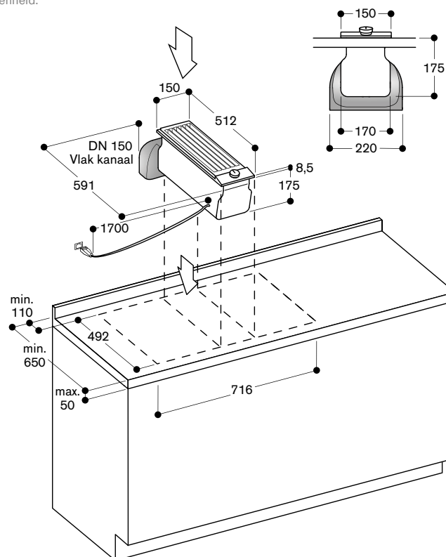
AD 410 040: Flexibel aansluitstuk voor de VL 200, DN 150 vlak.
