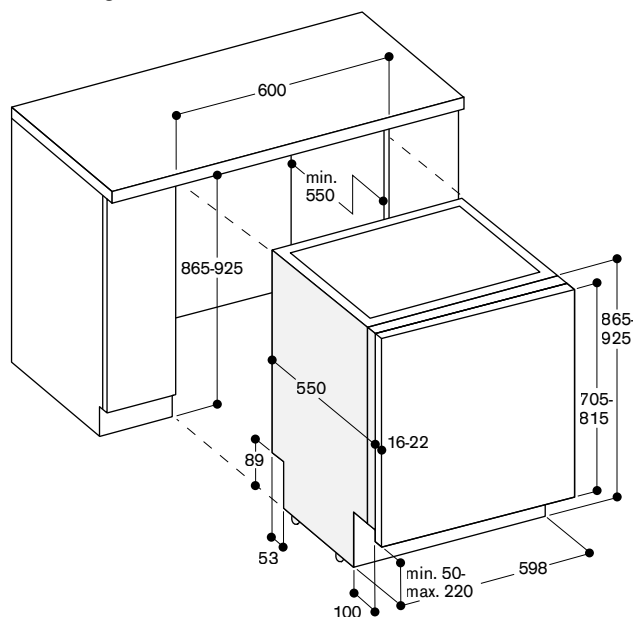
86,5 cm hogere vaatwasser met VarioScharnier
