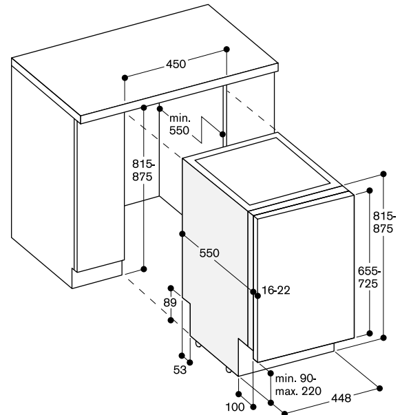
Aansluitmaten voor 45 cm brede afwasautomaat
