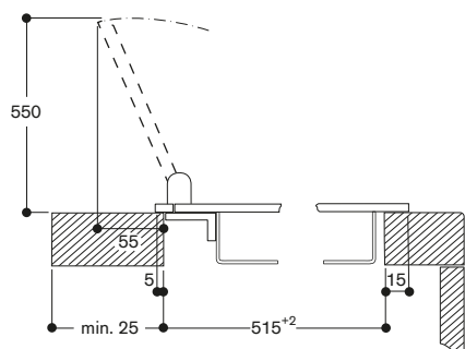
Installatie met deksel; Opbouw montage.
