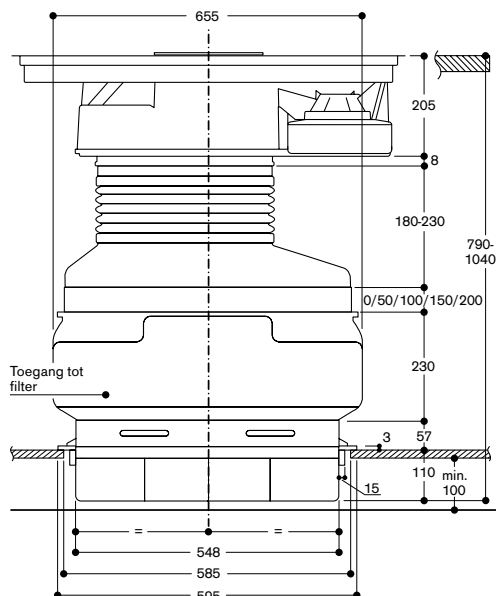
Vooraanzicht CV 282 met luchtcirculatiemodule CA 282 810
