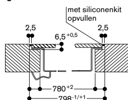
Langsdoorsnede
