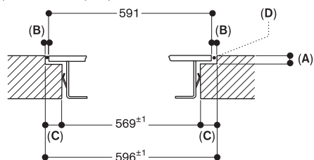
Продольный разрез
