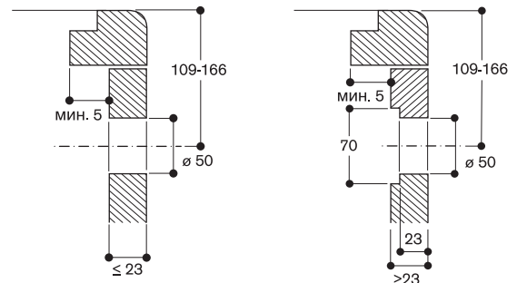
Встраиваемая в столешницу вытяжка VL 410
