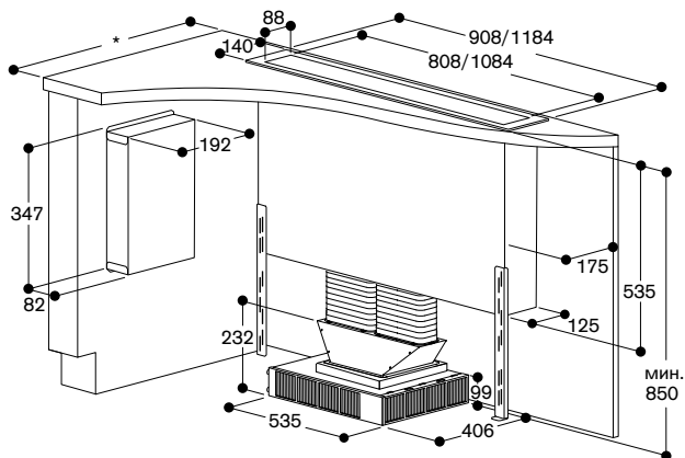
AL 400 с AR 413 122 (рециркуляция)
