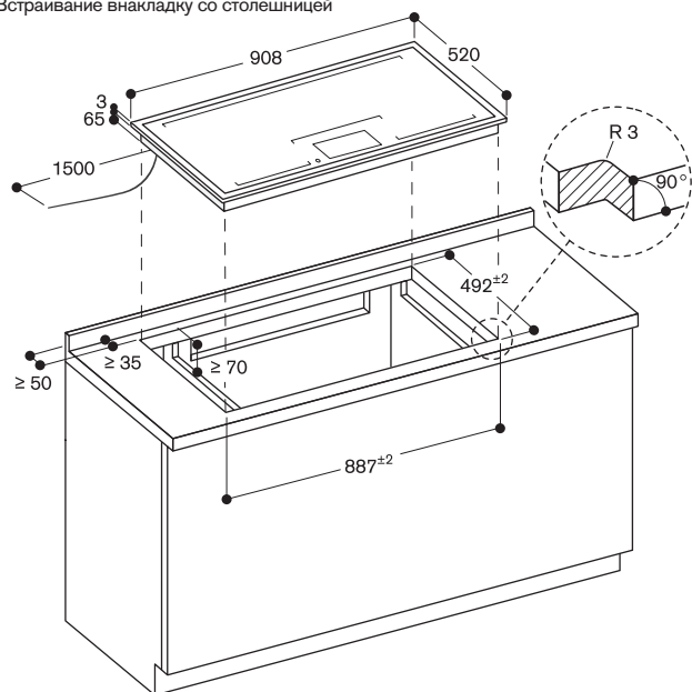
Встраивание внакладку со столешницей
