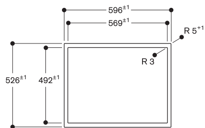
Вид сверху
