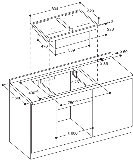
Вид спереди
