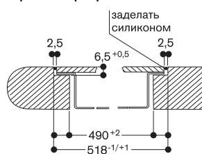
Поперечный разрез
