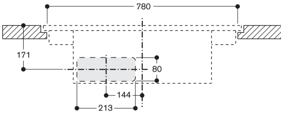
Вид спереди с CA 082 010
