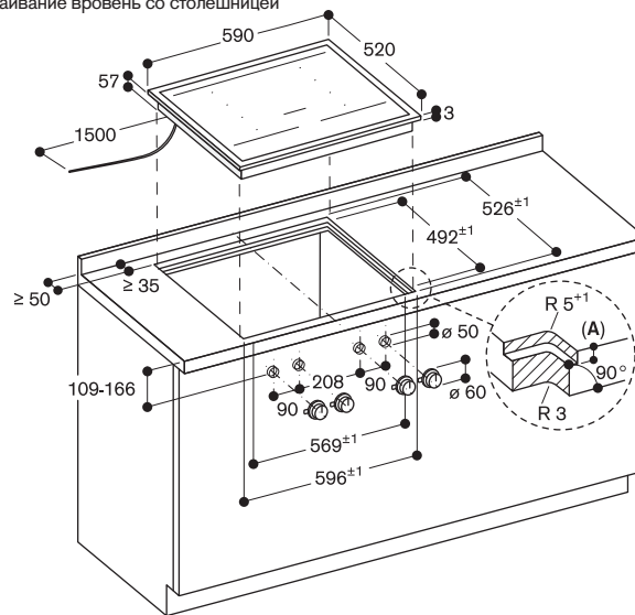
Встраивание вровень со столешницей
