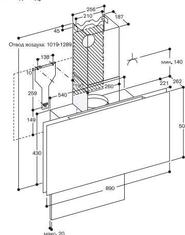
Отвод воздуха
