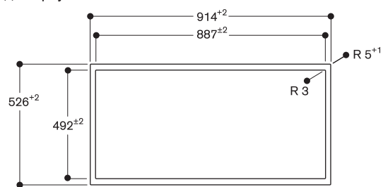
Вид сверху
