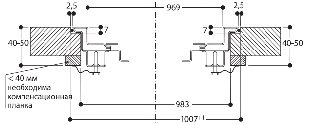
Продольный разрез
