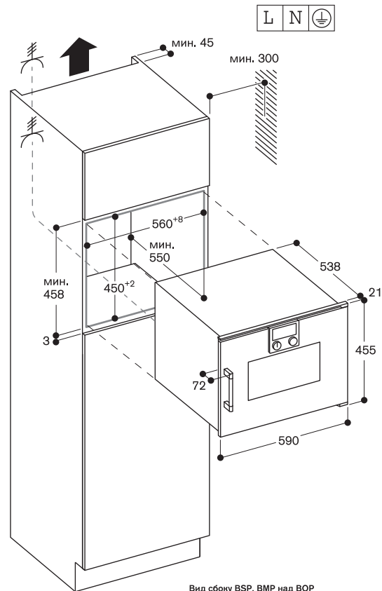
Вид сбоку BSP, BMP над BOP
