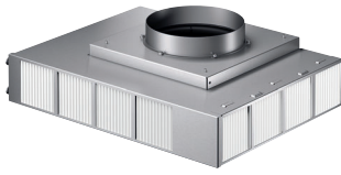
Вытяжной элемент серии 400 AR 413
