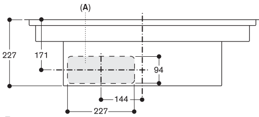
А: Подключается непосредственно к задней панели
