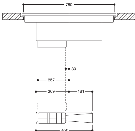
Вид спереди CV 282 с канальной рециркуляцией CA 082 020
