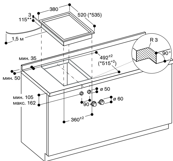
Установка внакладку со столешницей
