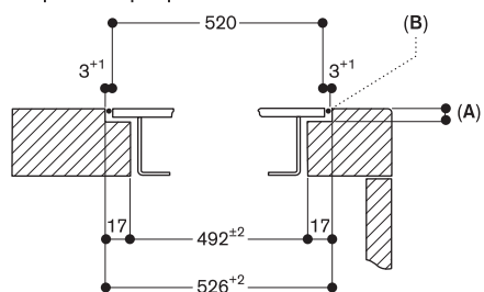
Поперечный разрез
