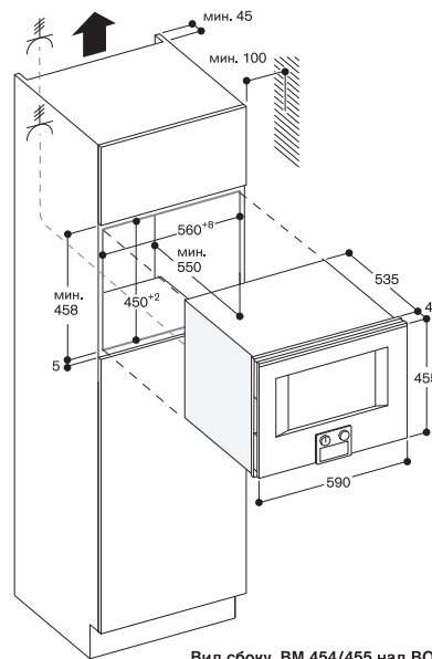
Вид сбоку, BM 454/455 над ВО
