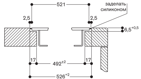
Поперечный разрез
