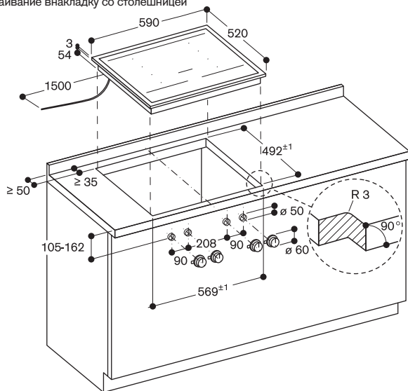
Встраивание внакладку со столешницей
