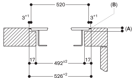
Поперечный разрез
