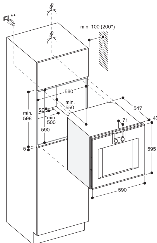
*200 мм вместе с BA 016
