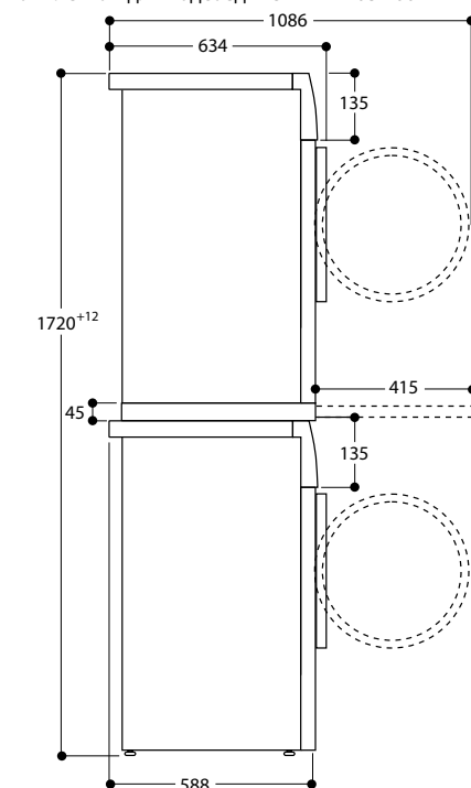
Вид сбоку, WT 260 под WM 260 с комплектом для подсоединения WA 032 001
