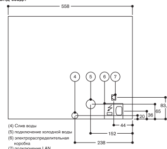
Вид сзади
