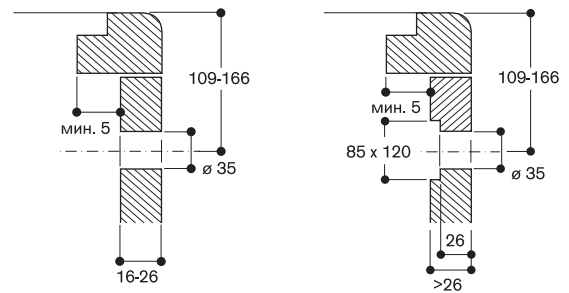
Встраиваемая в столешницу вытяжка VL 410
