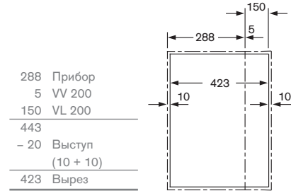
Размеры для монтажа Vario-приборов серии 200 со встраиваемой в столешницу вытяжкой
