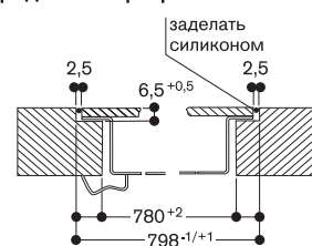
Продольный разрез
