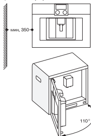
Встраивание в углу слева
