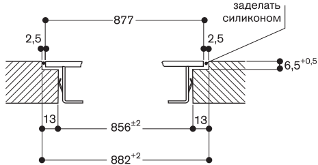
продольный разрез
