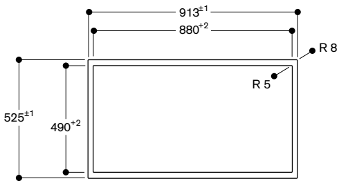
Вид сверху
