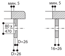
Монтаж переключателей
