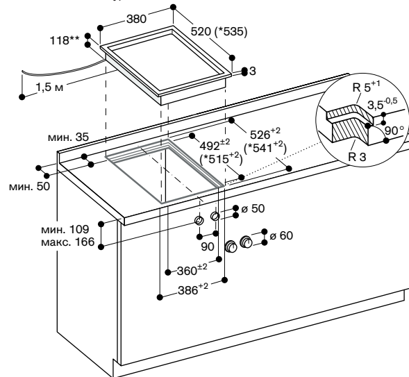
Установка на одном уровне со столешницей
