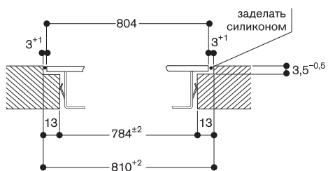
Продольный разрез
