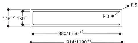
AL 400 вырез вровень с поверхностью
