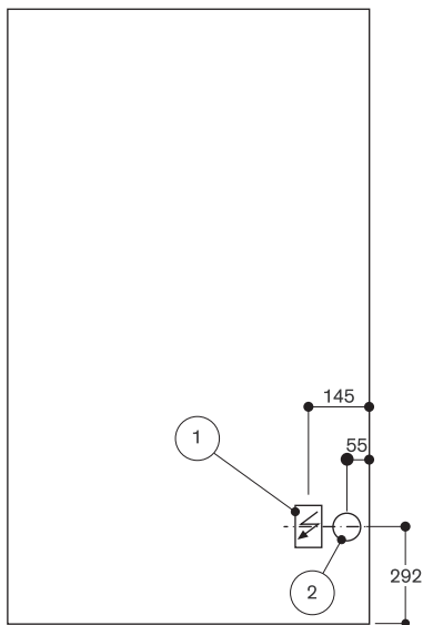
(1) разъем питания прибора (2) подключение прибора к водопроводу
