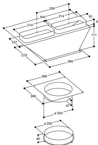
Mesures en mm
