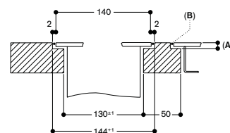
A: 3.5 ±0.5 mm B: Remplir avec du silicone
