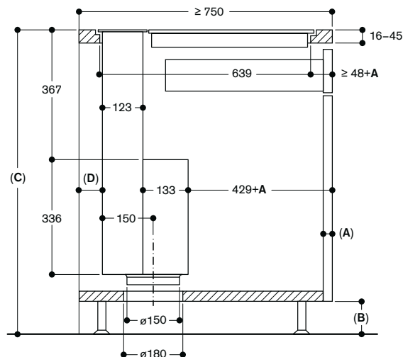
Vue latérale
