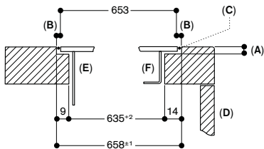
Coupe transversale
