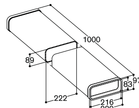
Mesures en mm
