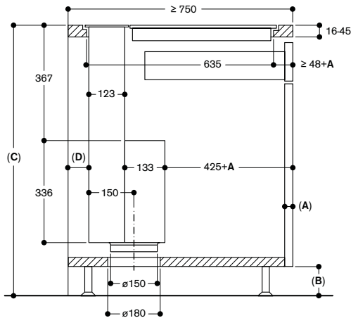
Vue latérale
