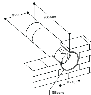
Mesures en mm
