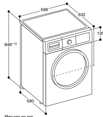
Mesures en mm
