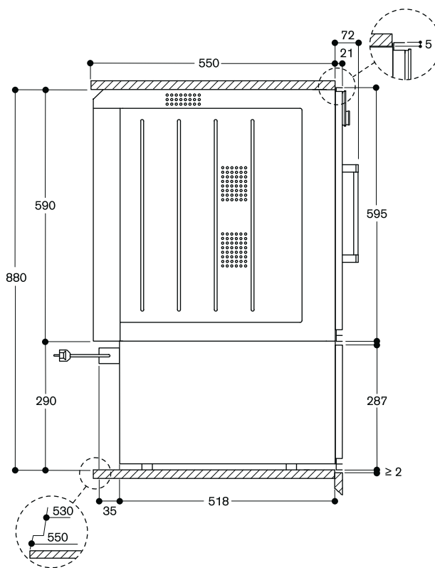
Mesures en mm
