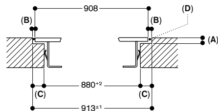
Coupe longitudinale
