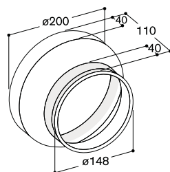
Mesures en mm
