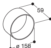
Mesures en mm
