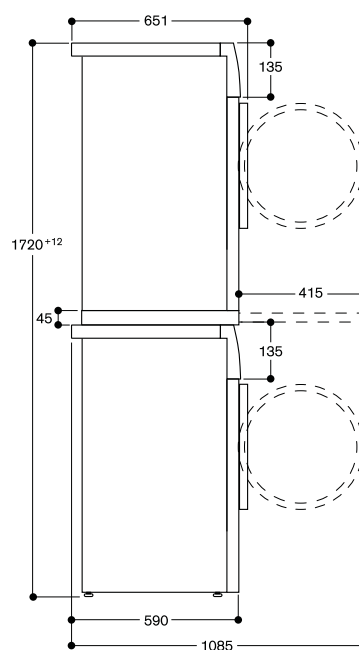
Mesures en mm
