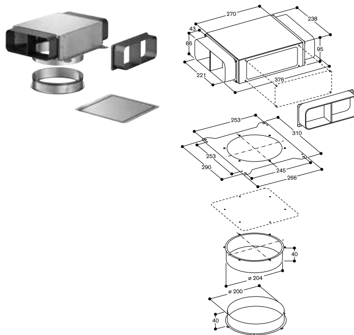
Mesures en mm
