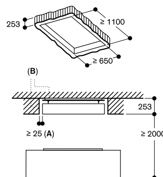
Mesures en mm
