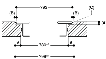
Coupe longitudinale
