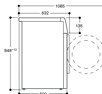
Mesures en mm
