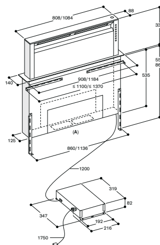
A : raccordement de la hotte à l'avant, à l'arrière ou par le bas
