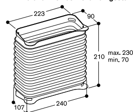
AD 410 040: Flexibel verbindingstuk voor VL200, DN 150 plat.
