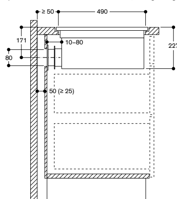
Zijaanzicht met kanaalloze recirculatie; vlak geïntegreerde inbouw
