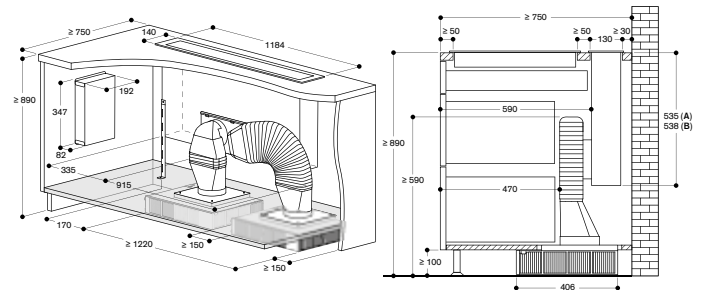
A: Inbouw met zichtbare rand B: Vlak geïntegreerde inbouw Afmeting in mm
