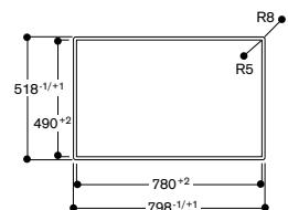
Aanzicht van boven
