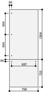
Nisbreedte 76,2 cm
