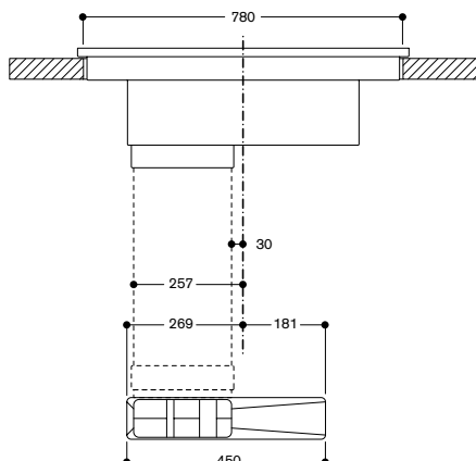
Vooraanzicht CV282 met gedeeltelijke geleide recirculatie set, inclusief diffuser (CA 082 061 / CA 082 071)
