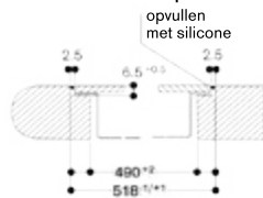
Doorsnede in de diepte
