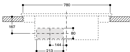
Vooraanzicht - meubeluitsnede voor kanaallose recirculatie; met zichtbare rand ingebouwd
