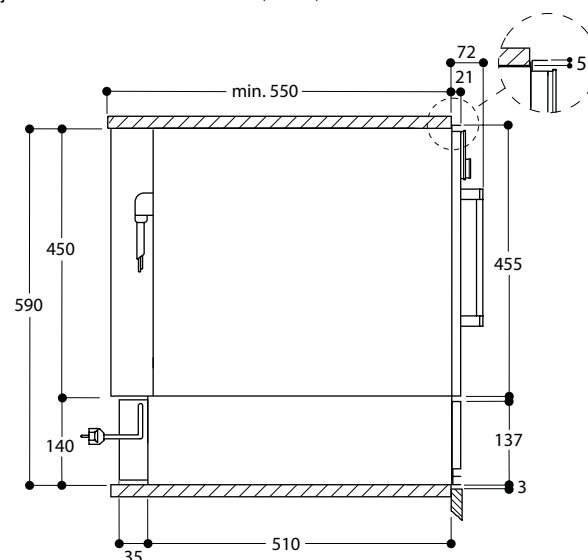
Zijaanzicht DVP 221 onder BSP, BMP, CMP
