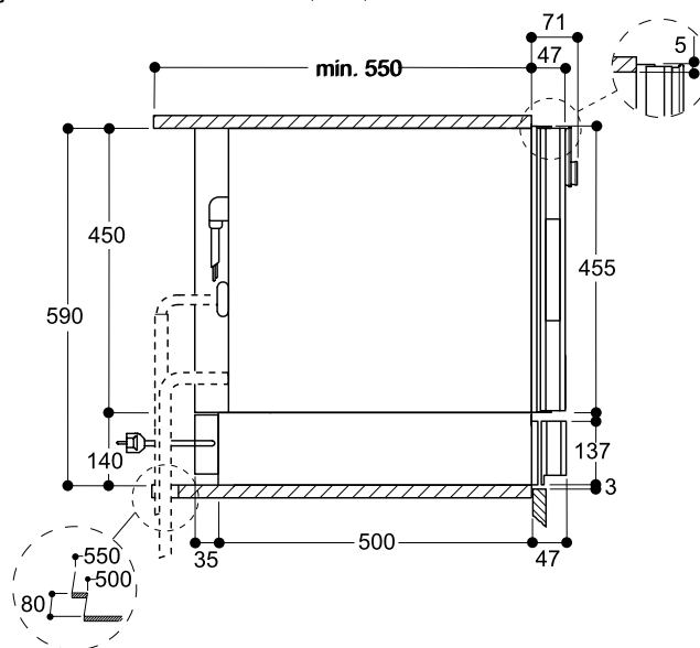
Zijaanzicht DV 461 onder BS, BM, CM
