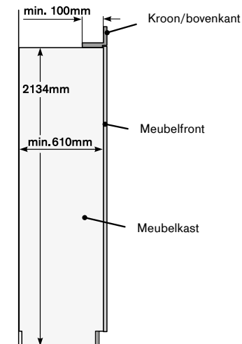
Zij-aanzicht installatie nis
