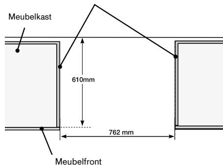
Boven-aanzicht installatie nis
