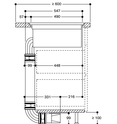
Zijaanzicht CV 282 met geleide recirculatie (CA 082 061)
