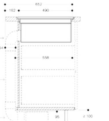
Zij aanzicht van de CV282 bij luchtafvoer. (CA 084 010)
