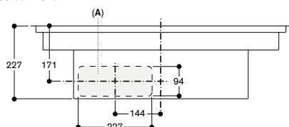
Vooraanzicht
