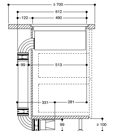
Zijaanzicht CV 282 met geleide recirculatie (CA 082 071)
