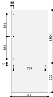
Nisbreedte 91,4 cm
