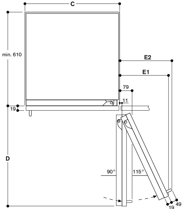
Wandafstand RB 472/RC/RF/RW
