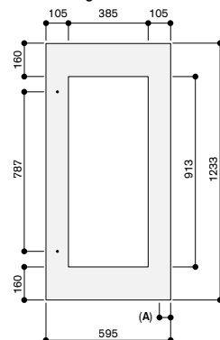
Front afmeting RW 222
