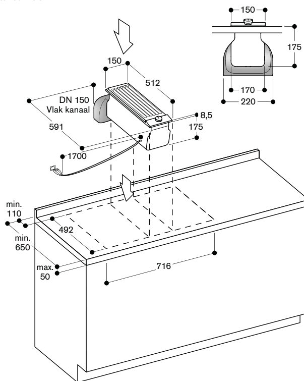
AD 410 040: Flexibel verbindingstuk voor VL200, DN 150 plat.
