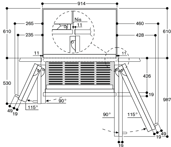
Wandafstand RB 492/RV 492
