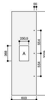
Nisbreedte 61 cm
