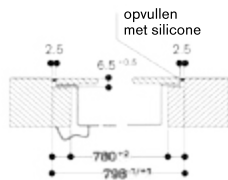
Doorsnede in de breedte
