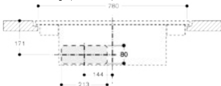
Afmetingen in mm
