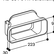
AD 851 041: Verbindingsstuk
