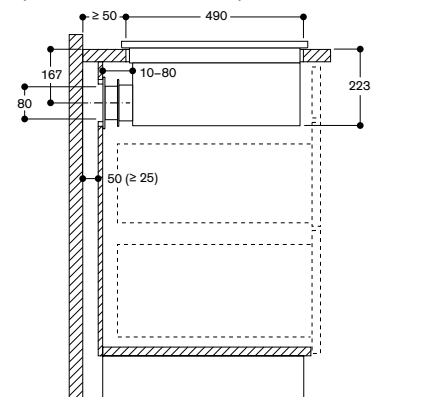
Zijaanzicht van de CV 282 met vrijblazende recirculatie CA 082 011
