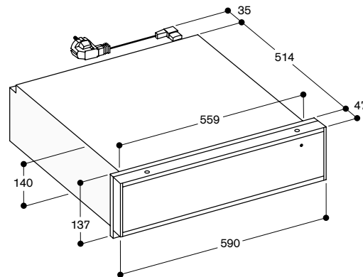
Afmeting in mm
