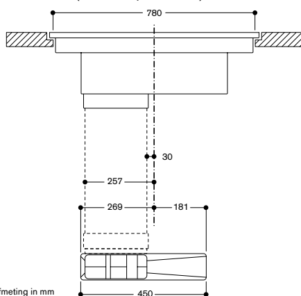
Vooraanzicht CV282 met gedeeltelijke geleide recirculatie set, inclusief diffuser (CA 082 061 / CA 082 071)
