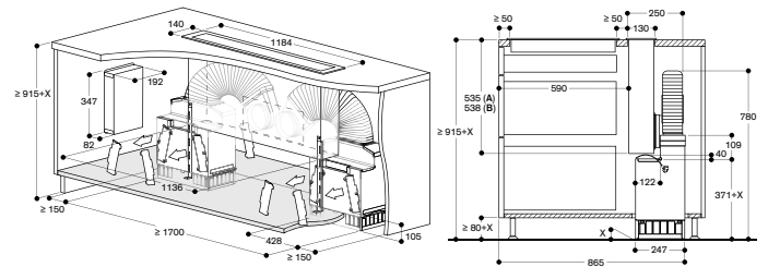
A: Inbouw met zichtbare rand B: Vlak geïntegreerde inbouw Afmeting in mm
