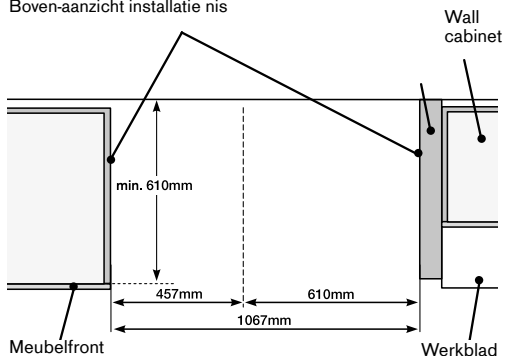
Boven-aanzicht installatie nis
