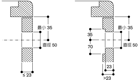
俯視圖
