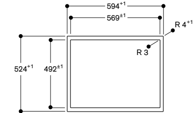
俯視圖
