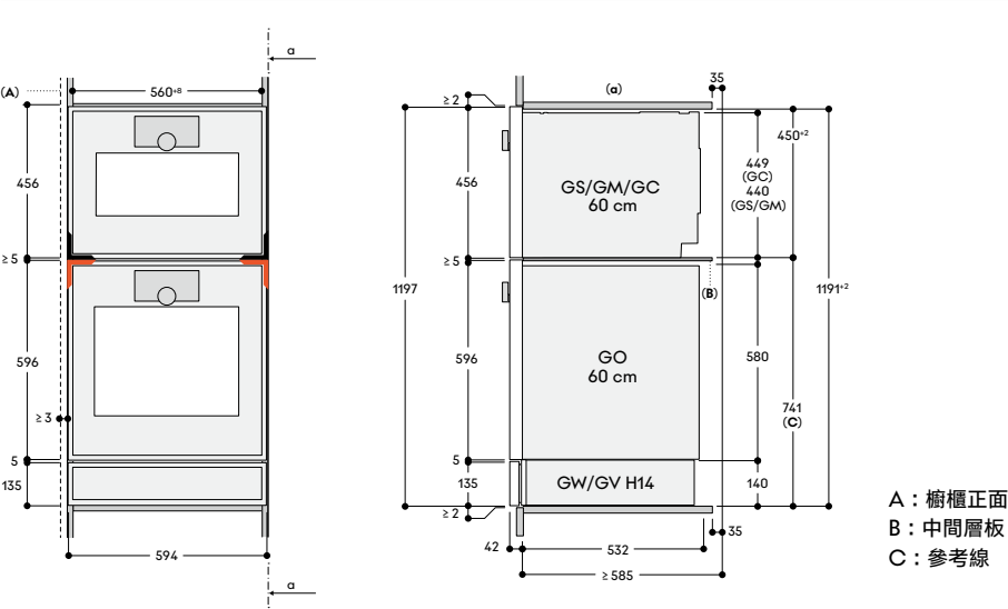
垂直組合-EV6_14_H45
