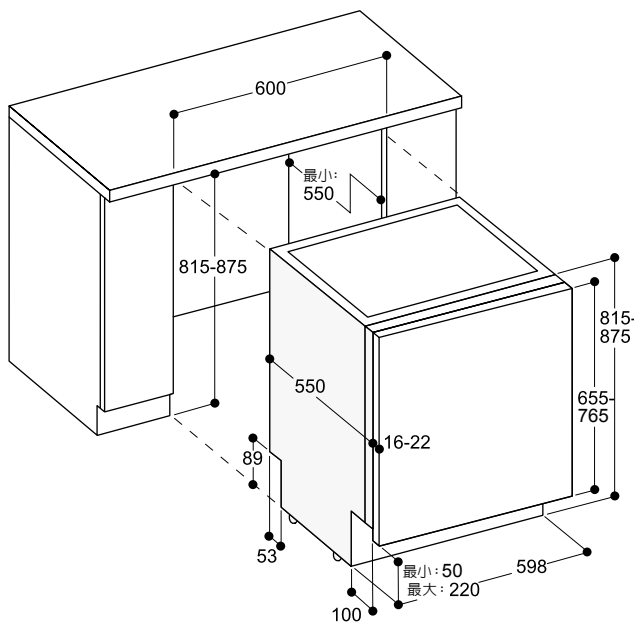
60 公分寬洗碗機的連接設計備註
