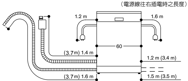
60 公分寬洗碗機的連接設計備註
