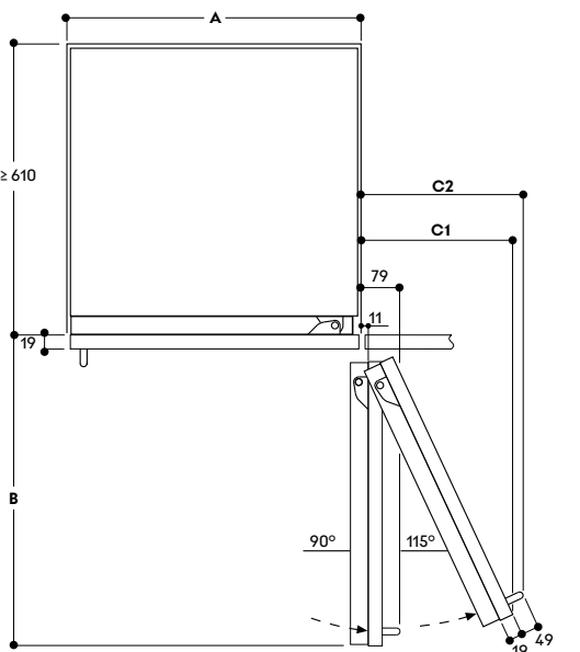
上圖中櫥櫃門板厚度為19mm，Gaggenau 冰箱把手高度為49mm A:610 B:677 C1:299 C2:330
