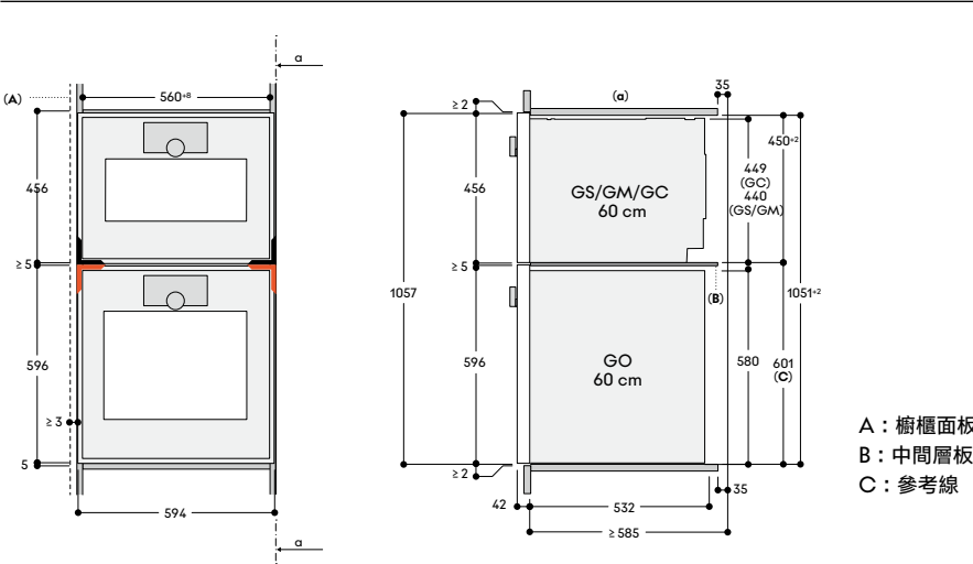
垂直組合-EV6_0_H45 GA 601 010 中間層板
