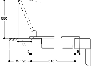
加裝不鏽鋼爐蓋：上裝安裝
