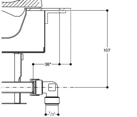
連接瓦斯
