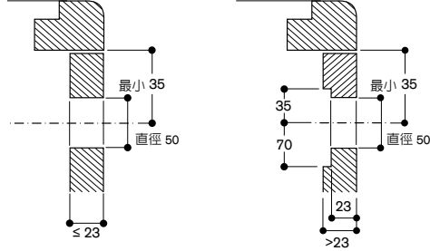
控制旋鈕安裝縱剖面圖：平接安裝
