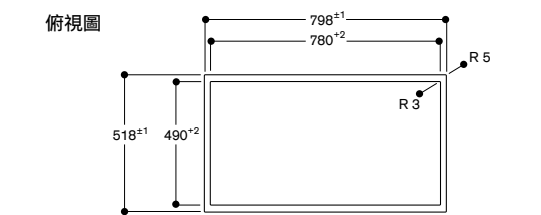
A: 6.5+0.5 B: 若檯面超過600mm請參照安裝手冊
