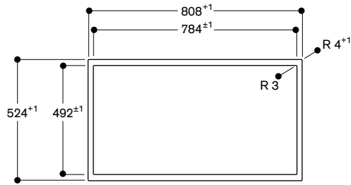
俯視圖
