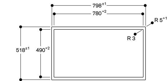
俯視圖
