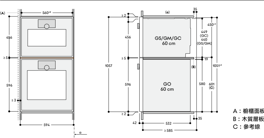
垂直組合-EV6_0_H45 木質層板
