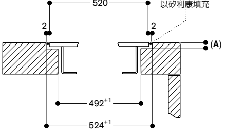
縱剖圖
