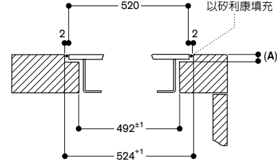
縱剖圖
