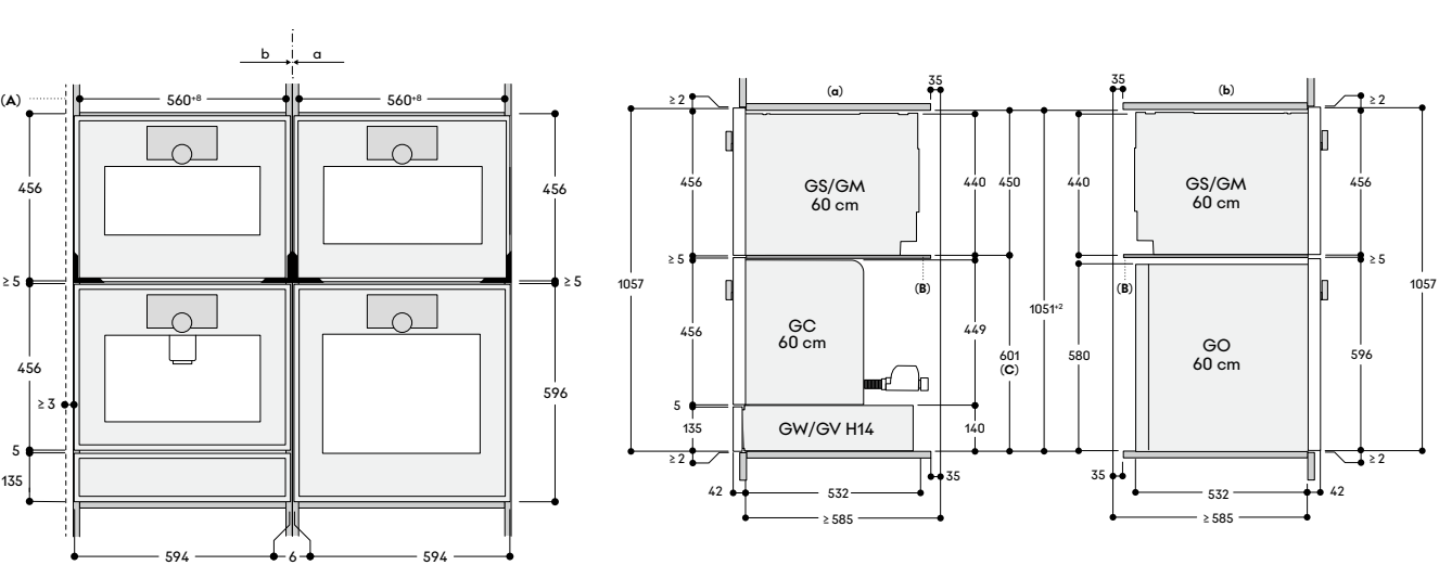
四宮格組合-ECU66_14_H45
