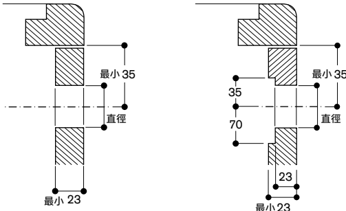
控制旋鈕的安裝：平接安裝
