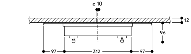
橫剖圖
