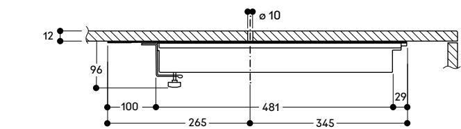
縱剖圖
