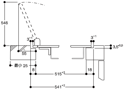
加裝不鏽鋼爐蓋：上裝安裝
