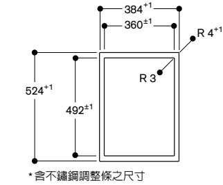
橫剖圖
