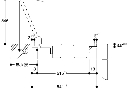
加裝不鏽鋼爐蓋：上裝安裝
