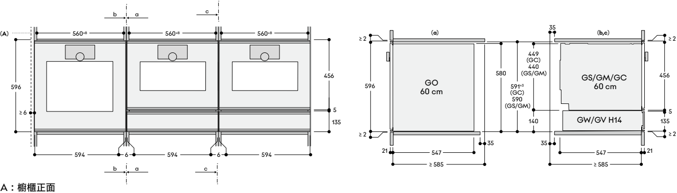
A：櫥櫃正面
