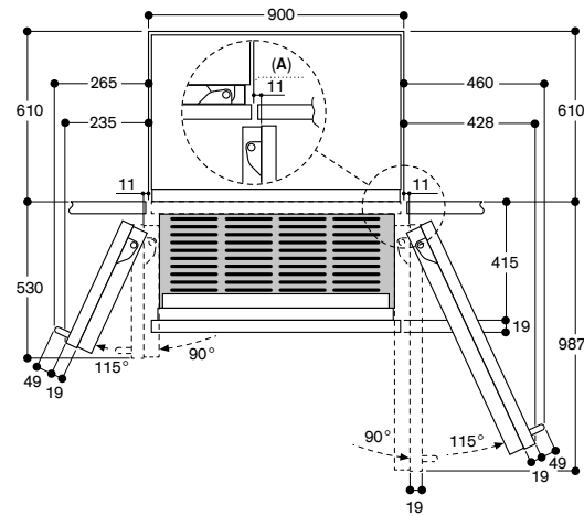
A：內縮 上圖中櫥櫃門板厚度為19mm，Gaggenau 冰箱把手高度為49mm
