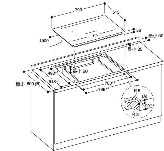
A: 6.5+0.5 B: 若檯面超過600mm請參照安裝手冊
