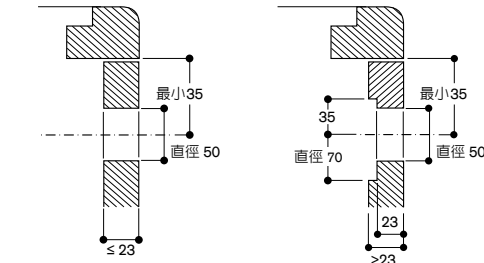
控制旋鈕安裝縱剖圖；平接安裝
