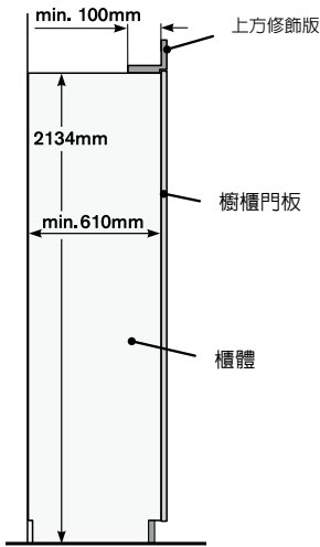
側視圖：
