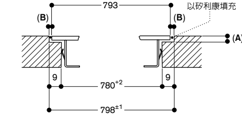
縱剖面
