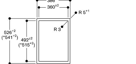
俯視圖
