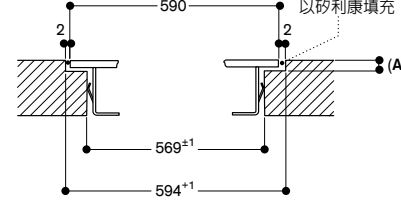
橫剖圖
