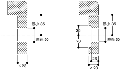
控制旋鈕安裝縱剖面圖：上裝安裝
