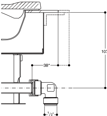
加裝不鏽鋼爐蓋：平接安裝
