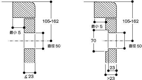
連接瓦斯
