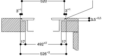
縱剖圖
