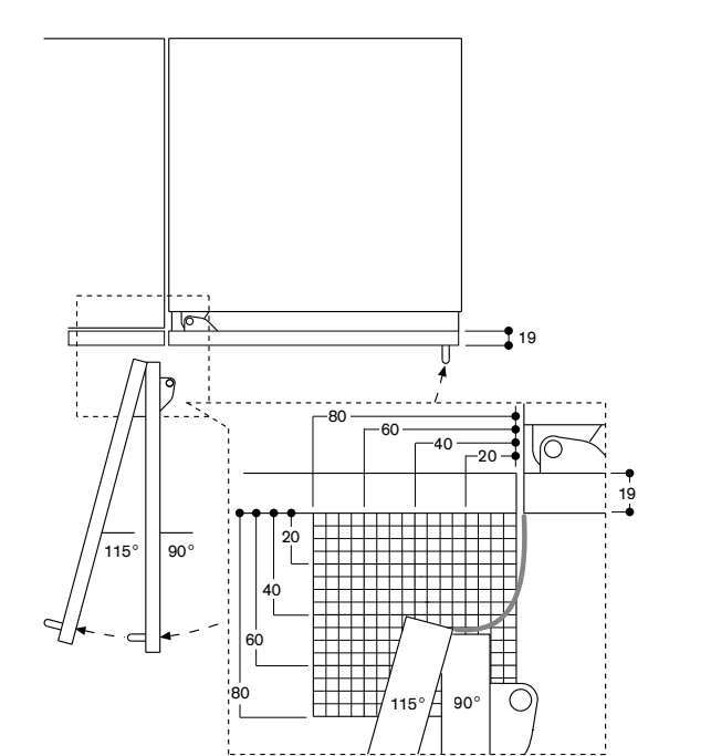
上圖標示鉸鍊旋轉空間與相連櫥櫃的相應距離。圖中櫥櫃門板厚度為19mm
