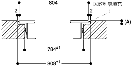
橫剖圖
