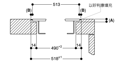
橫剖面
