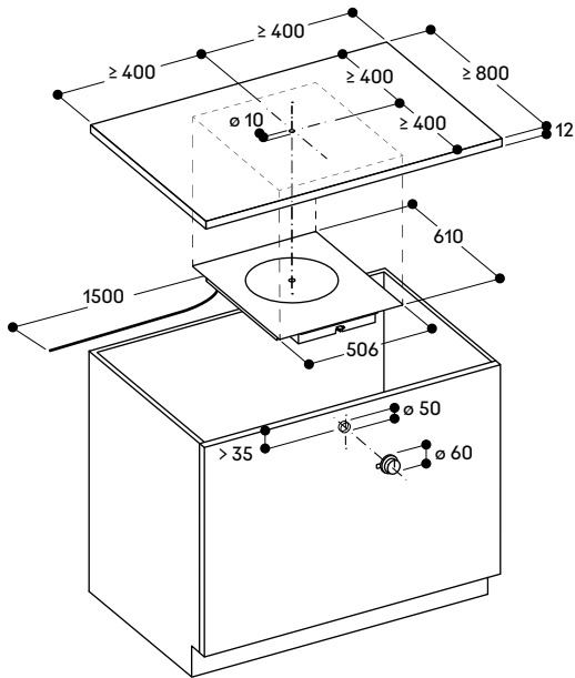
俯視圖
