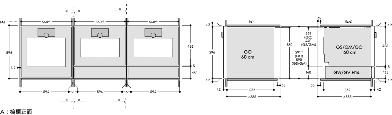
水平組合-EH66_14
