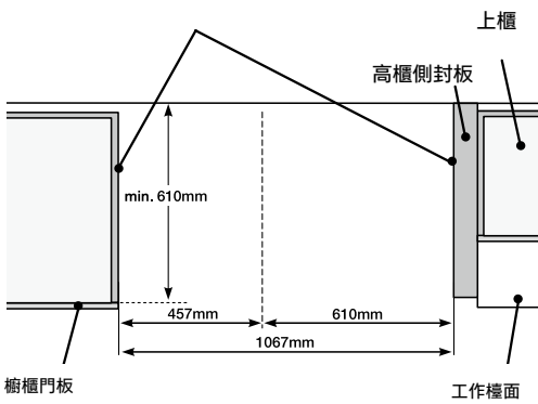
水平俯視
