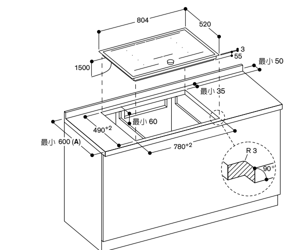
A: 若檯面超過600mm請參照安裝手冊
