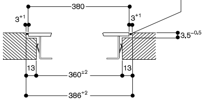
縱剖圖
