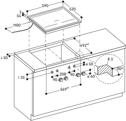
Montage Kochfeld; aufgesetzter Einbau
