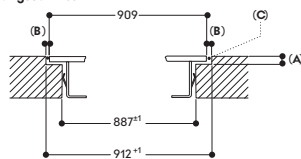
Längsschnitt
