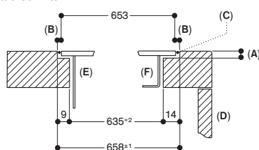
Querschnitt
