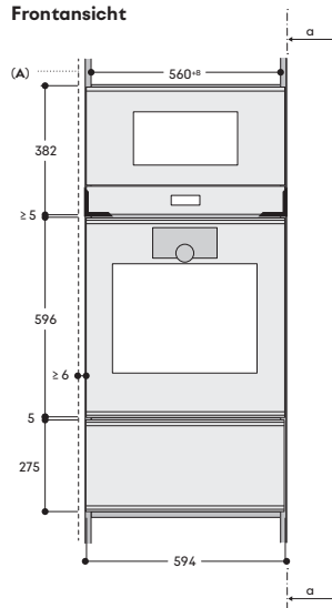
Frontansicht
