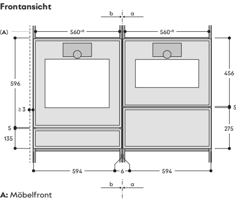
A: Möbelfront
