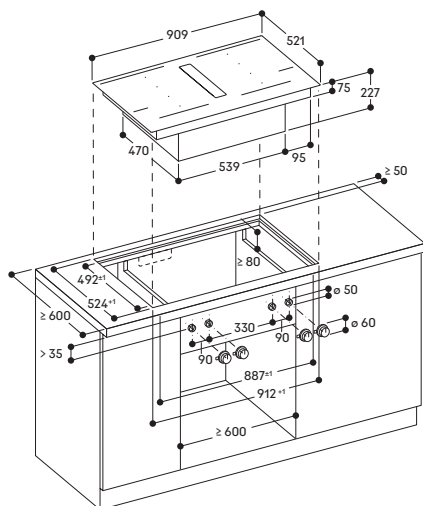
Montage Kochfeld; flächenbündiger Einbau
