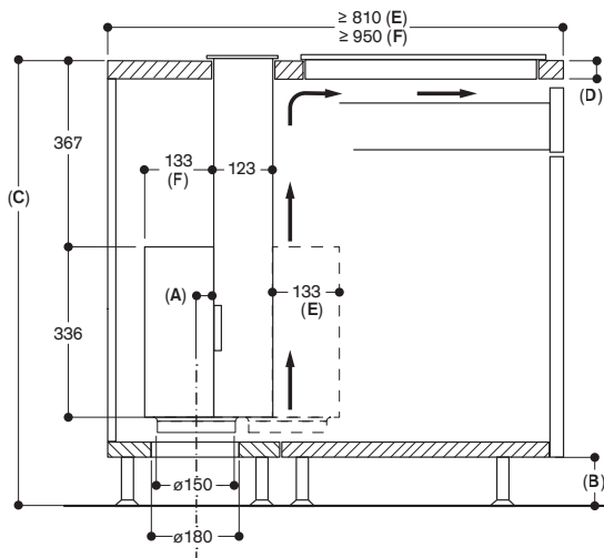
Seitenansicht
