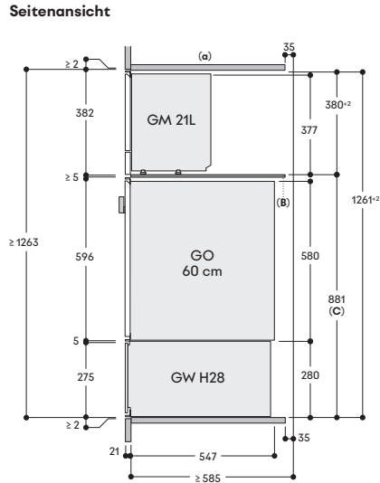
Seitenansicht
