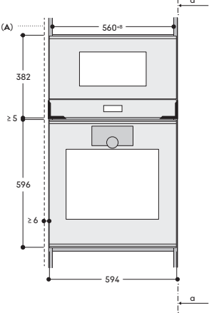
Frontansicht
