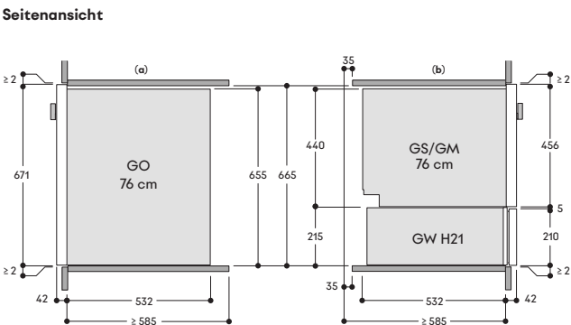
Seitenansicht
