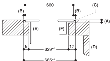
Querschnitt
