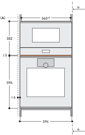
Frontansicht
