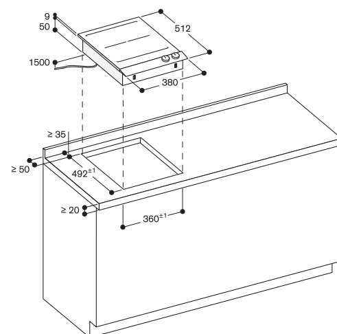
Montage Kochfeld; aufgesetzter Einbau
