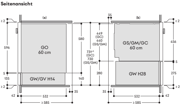
Seitenansicht
