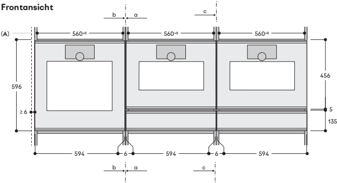
A: Möbelfront
