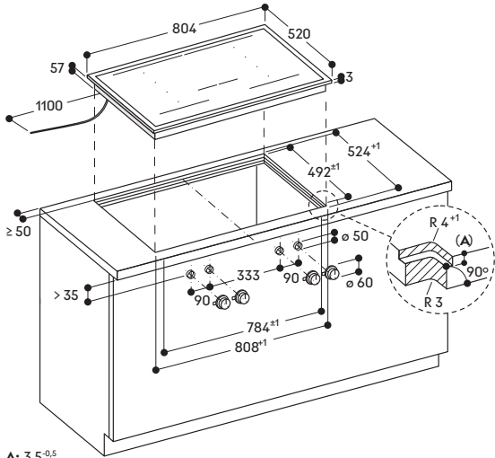
Montage Kochfeld; flächenbündiger Einbau
