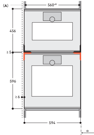
Frontansicht
