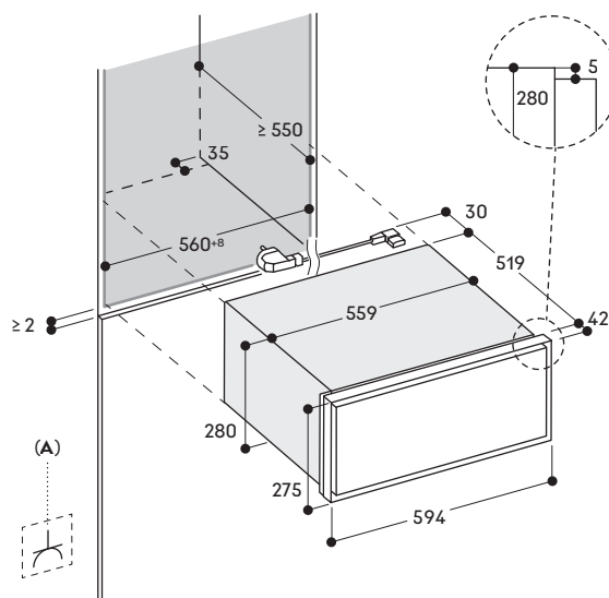
A: Frei zugänglicher elektrischer Anschluss
