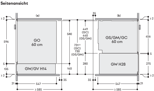
Seitenansicht
