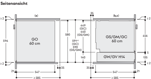
Seitenansicht
