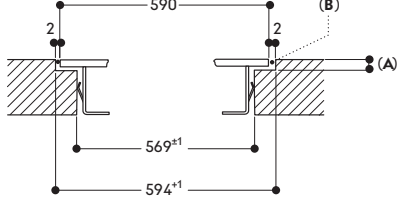
Längsschnitt
