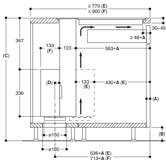
Seitenansicht
