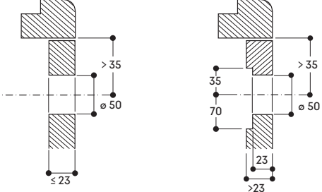
Montage Bedienknebel
