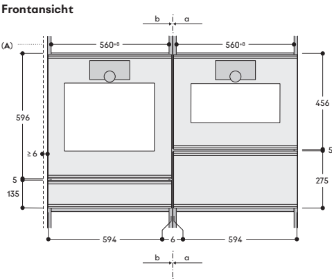
A: Möbelfront
