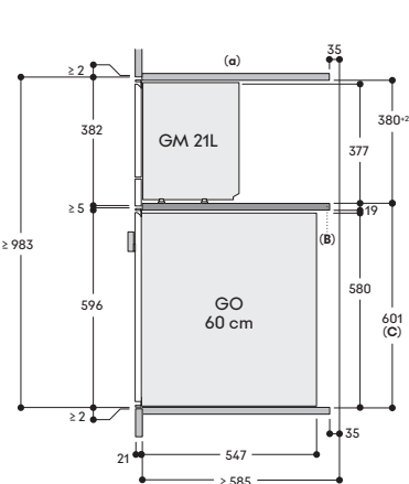
Seitenansicht
