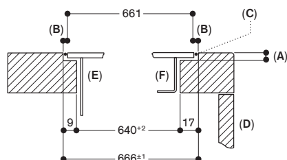
Querschnitt
