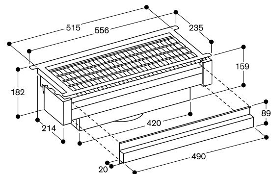
abnehmbare Filterblende
