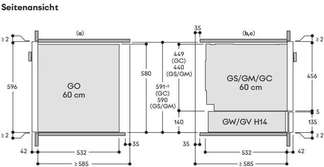
Seitenansicht
