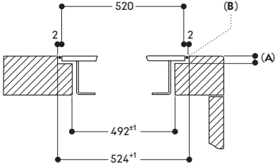
Querschnitt
