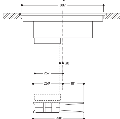
Vorderansicht von CV 492 mit ungeführter Umluft.
