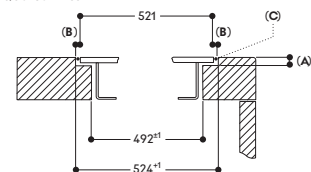
Querschnitt
