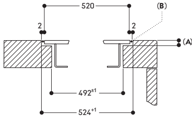
Querschnitt
