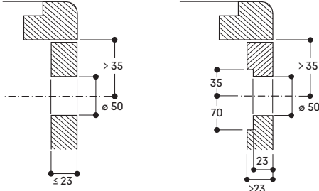
Montage Bedienknebel
