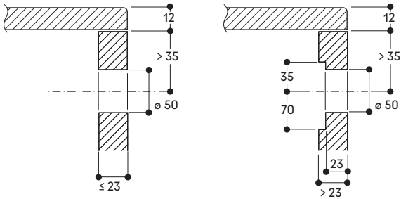
Montage Bedienknebel
