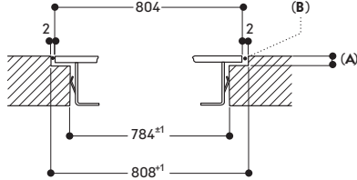
Längsschnitt
