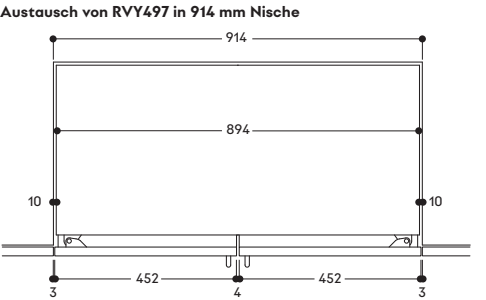
Die resultierenden seitlichen Spalten von 10 mm können mit den Seitenblenden verkleidet werden, die im Installationszubehör RVA460910 enthalten sind.
