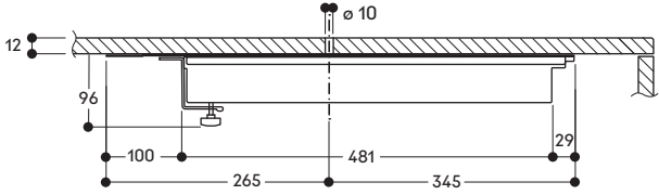
Längsschnitt
