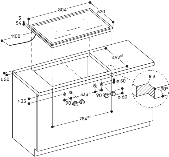
Montage Kochfeld; aufgesetzter Einbau
