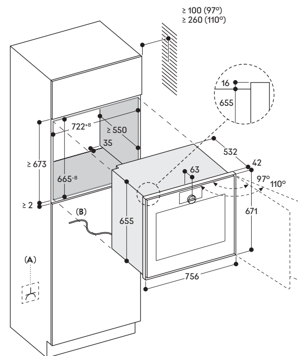
A: Frei zugänglicher elektrischer Anschluss B: Fest eingebautes Kabel
