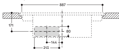
Vorderansicht - Möbelausschnitt für ungeführte Umluft - flächenbündig.
