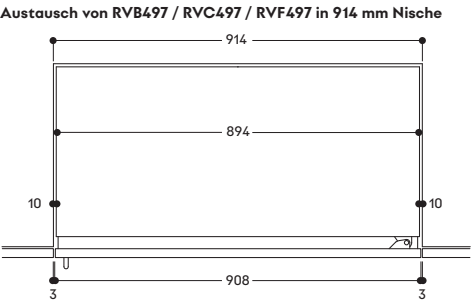
Die resultierenden seitlichen Spalte von 10mm können mit den Seitenblenden verkleidet werden, die im Installationszubehör RVA460910 enthalten sind
