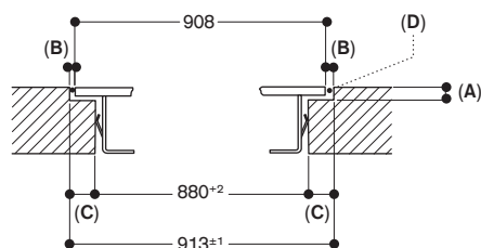
Längsschnitt
