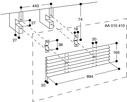
AA 010 410 Luftauslassgitter
