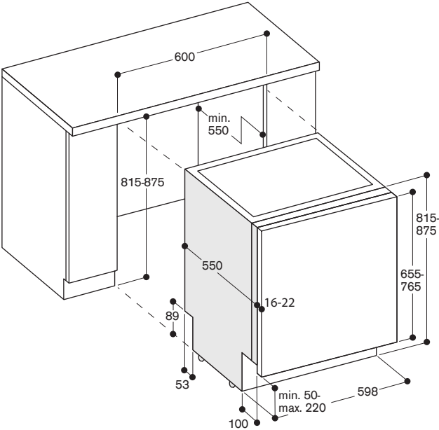
81,5 cm hoher Geschirrspüler mit flexiblem Scharnier
