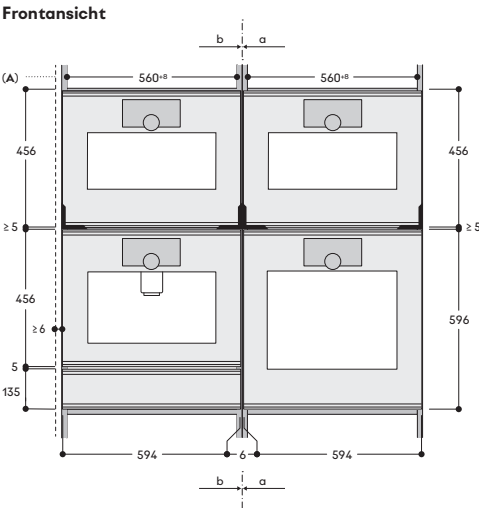
A: Möbelfront
