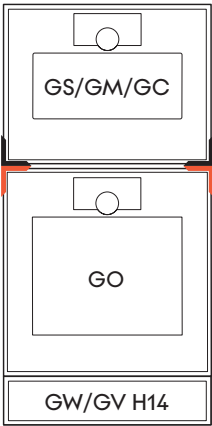
Kombination EV6_14_H45 (Abmessungen, siehe Seite 16)
