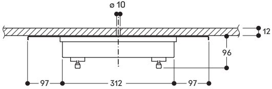
Querschnitt
