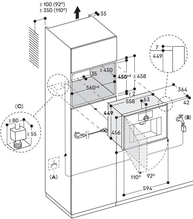
A: Frei zugänglicher elektrischer Anschluss B: Frei zugänglicher Wasseranschluss C: Zusätzlicher Ausschnitt für Aquastop
