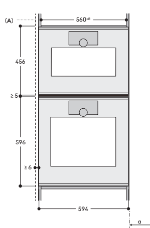
Frontansicht
