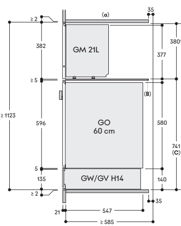
Seitenansicht
