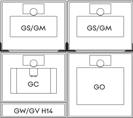
Kombination ECU66_14_H45 (Abmessungen, siehe Seite 19)
