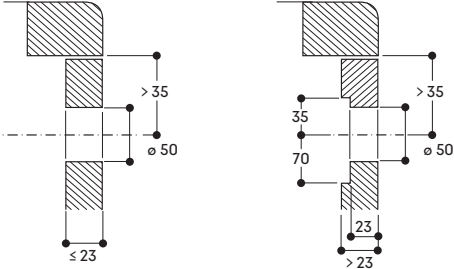
Montage Bedienknebel
