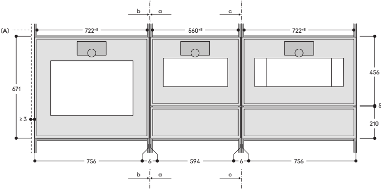
Seitenansicht
