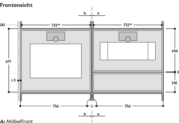
A: Möbelfront
