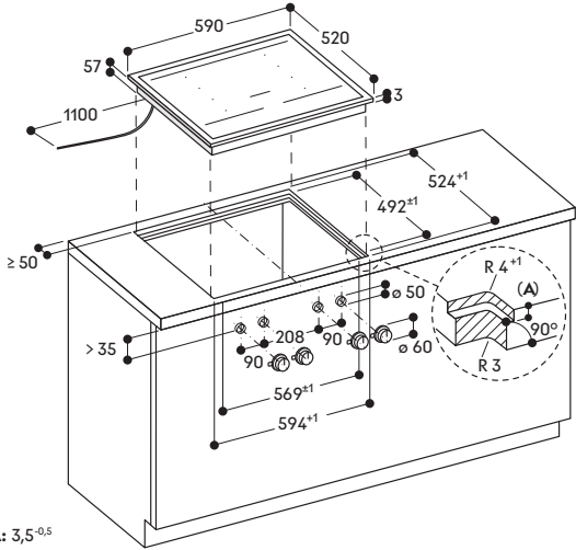
Montage Kochfeld; flächenbündiger Einbau
