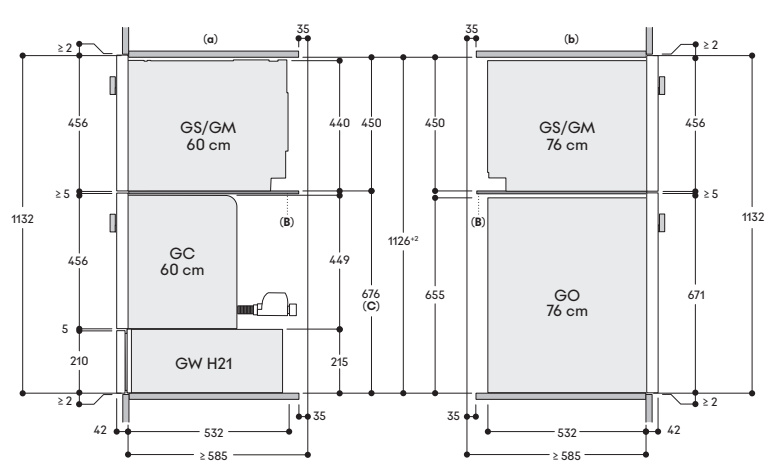
Seitenansicht
