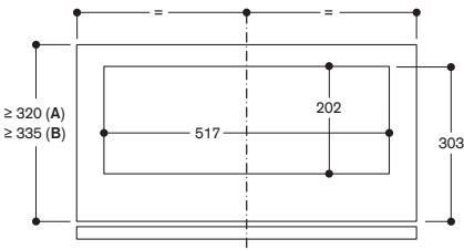
Ansicht von Oberschrank von oben mit AA 211 812
