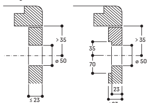
Montage Bedienknebel
