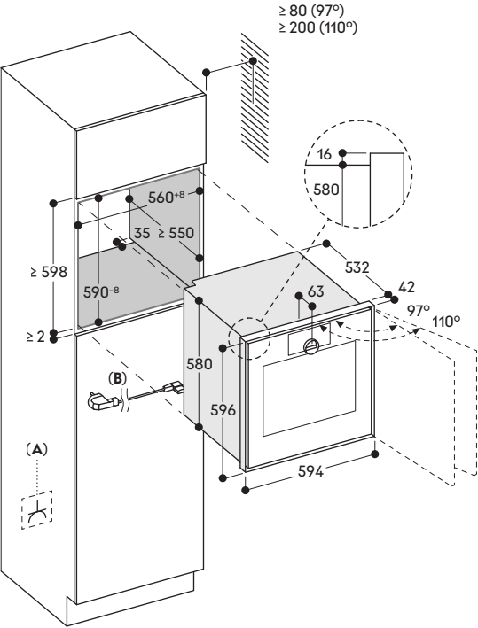
A: Frei zugänglicher elektrischer Anschluss B: Kabel mit oder ohne Stecker, je nach Land
