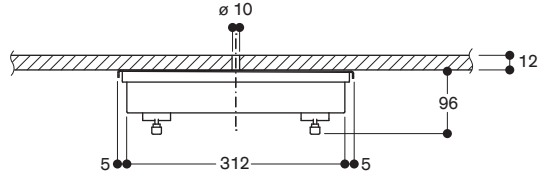
Querschnitt
