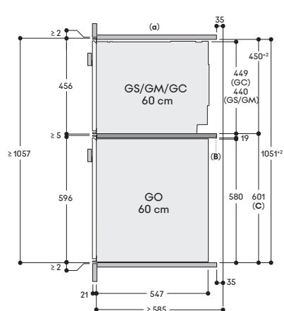
Seitenansicht
