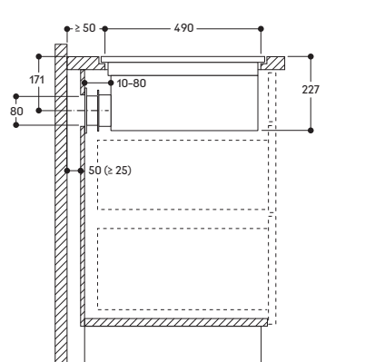
Seitenansicht mit ungeführter Umluft; flächenbündiger Einbau
