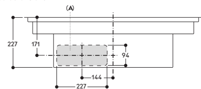
Vorderansicht
