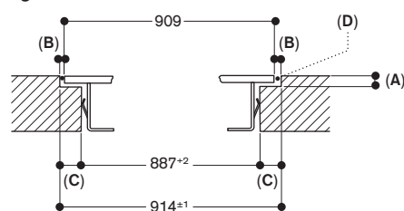
Längsschnitt
