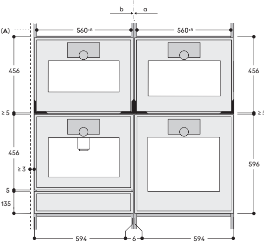
Frontansicht
