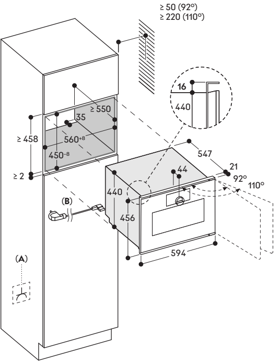
A: Frei zugänglicher elektrischer Anschluss B: Kabel mit oder ohne Stecker, je nach Land
