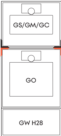
Kombination EV6_28_H45 (Abmessungen, siehe Seite 17)
