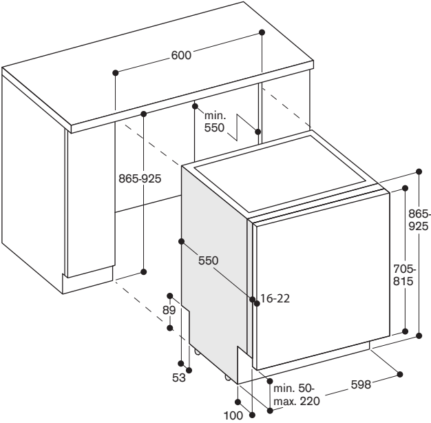
86,5 cm hoher Geschirrspüler mit flexiblem Scharnier
