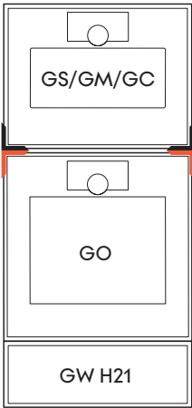
Kombination EV6_21_H45 (Abmessungen, siehe Seite 17)
