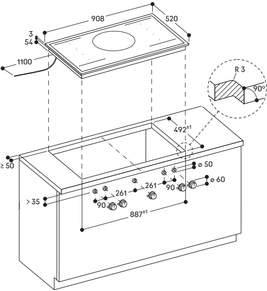
Montage Kochfeld; aufgesetzter Einbau
