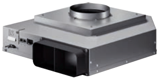
Gebläsebaustein AR403
