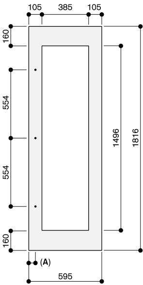
Höhe der Aussparung 178 cm
