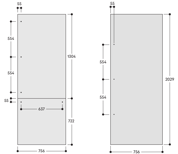
Nischenbreite 762 mm
