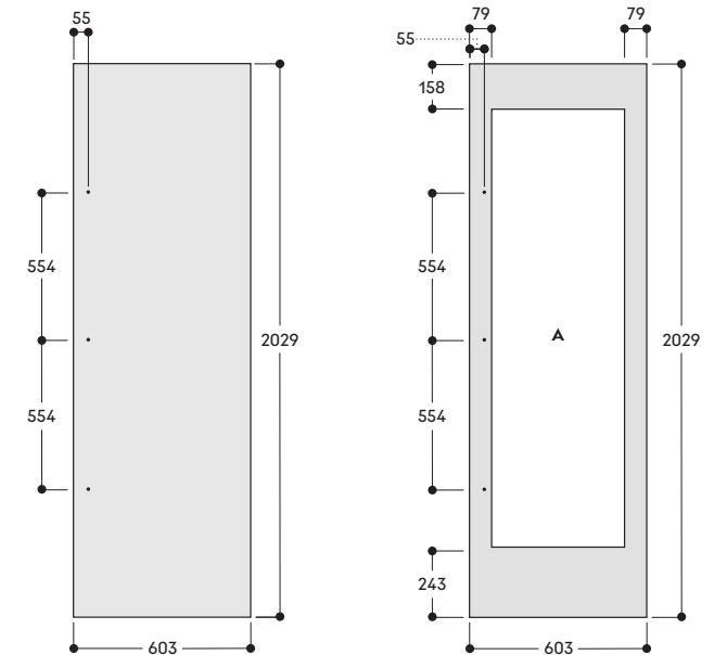
Nischenbreite 610 mm
