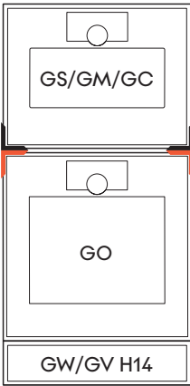
Kombination EV6_14_H45 (Abmessungen, siehe Seite 16)
