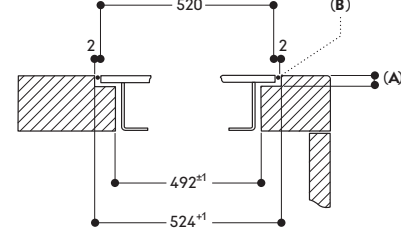
Querschnitt
