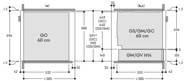
Seitenansicht
