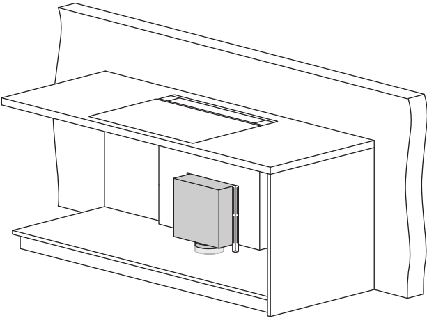
Planungsbeispiel — Gebläsebaustein an der Vorderseite
