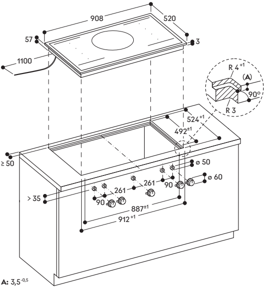
Montage Kochfeld; flächenbündiger Einbau
