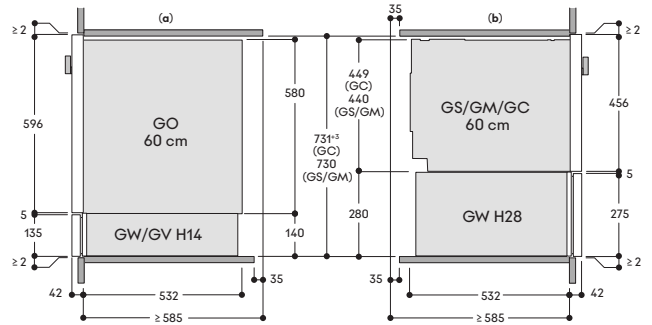
Seitenansicht
