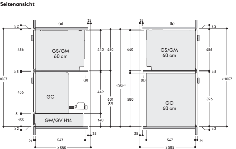
Seitenansicht
