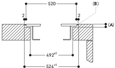
Querschnitt
