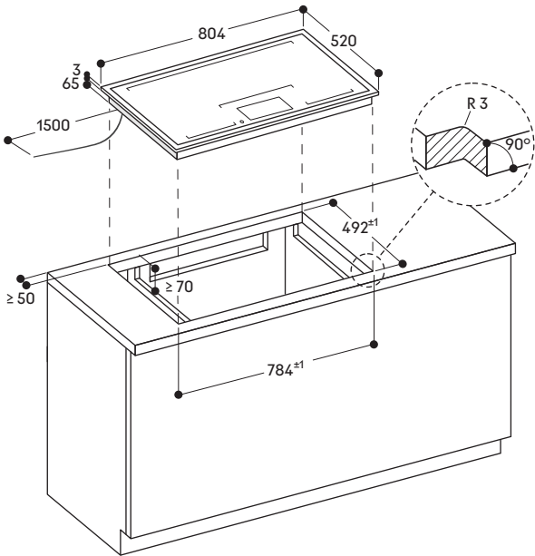
Montage Kochfeld; aufgesetzter Einbau
