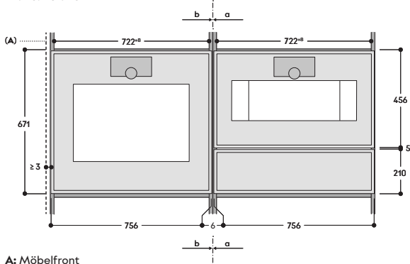
A: Möbelfront
