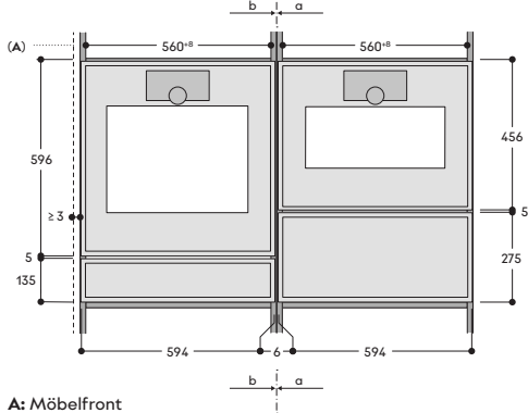
A: Möbelfront
