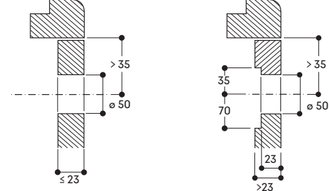
Montage Bedienknebel
