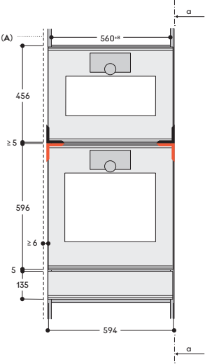
Frontansicht
