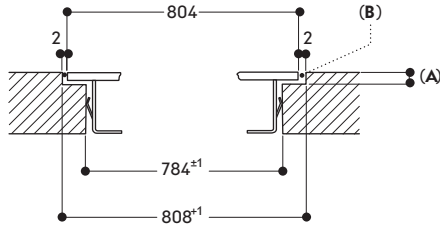
Längsschnitt
