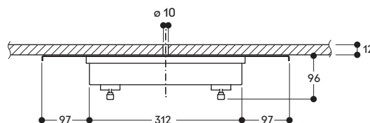
Querschnitt
