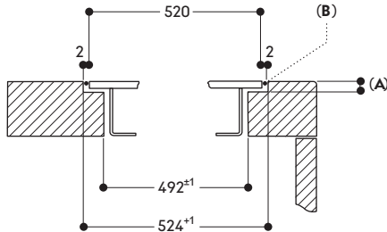
Querschnitt
