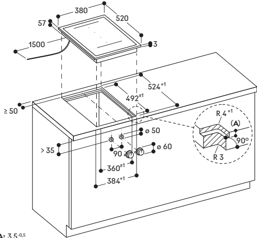
Montage Kochfeld; flächenbündiger Einbau
