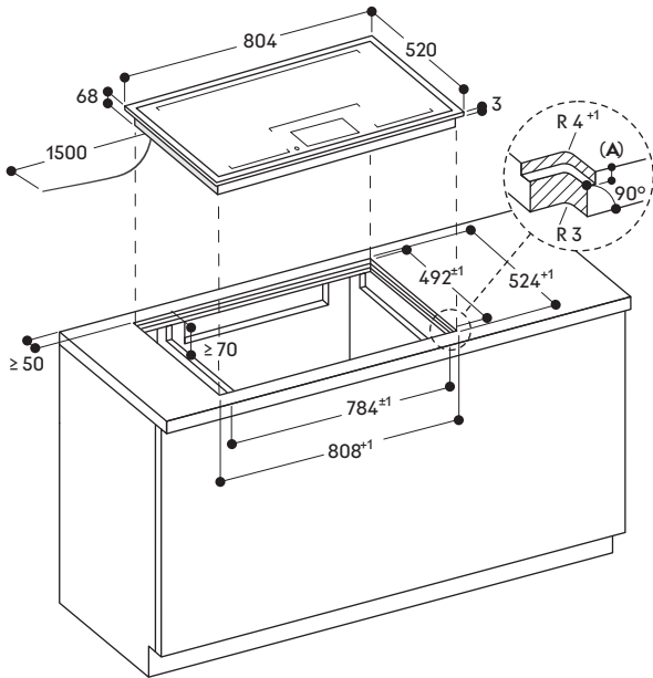
Montage Kochfeld; flächenbündiger Einbau
