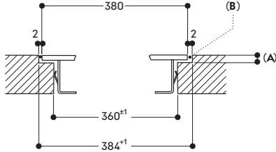
Längsschnitt
