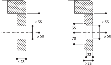
Montage Bedienknebel
