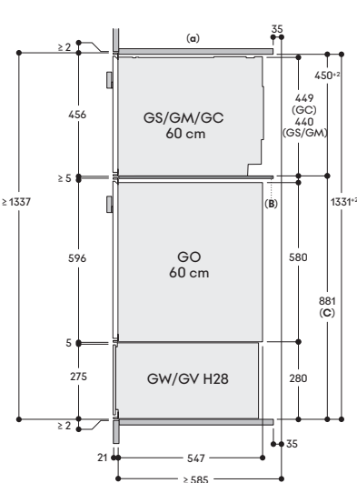
Seitenansicht
