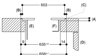
Querschnitt
