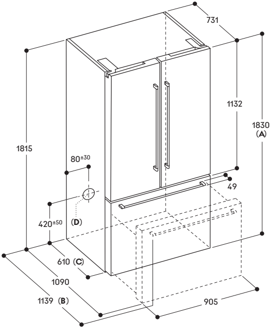
Vista apparecchio tridimensionale e dimensioni nicchia
