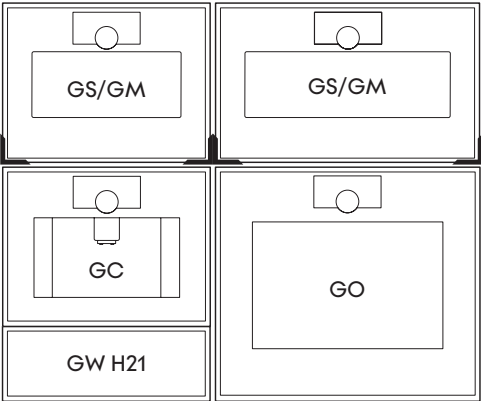
Combinazione ECU63_21_H45 (Dimensioni, vedi pagina 23)
