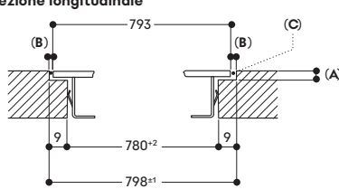
Sezione longitudinale
