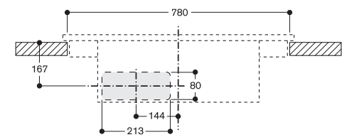
Vista frontale - foro d'incasso per ricircolo non canalizzato
