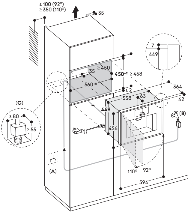
A: Presa elettrica B : Connessione alla rete idrica C: Taglio aggiuntivo per il passaggio dell'Aquastop
