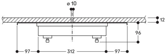
Sezione trasversale
