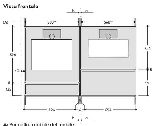
A: Pannello frontale del mobile
