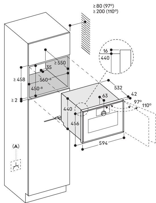
A: Presa elettrica
