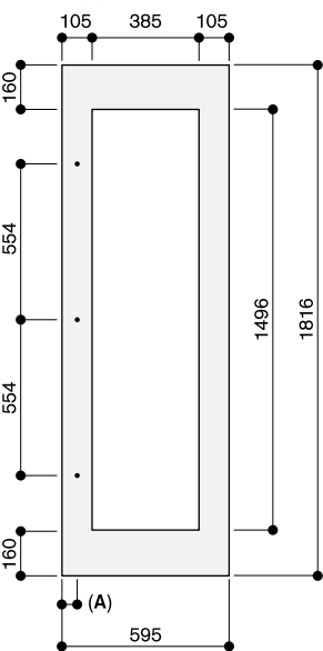
Altezza apparecchio 178 cm
