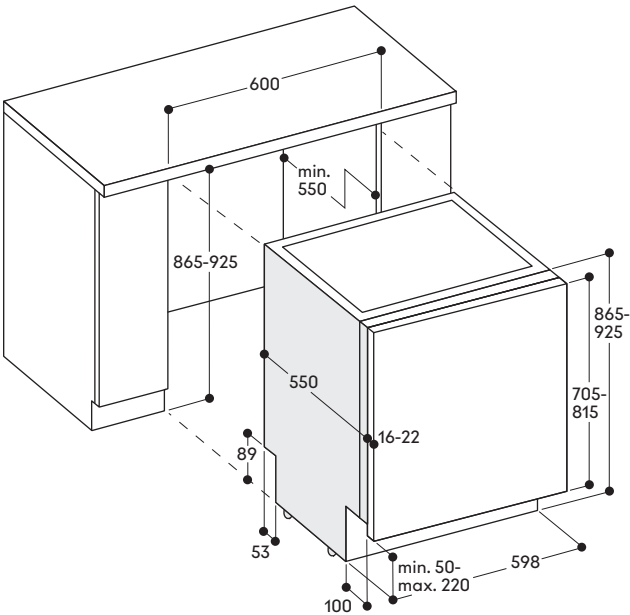
Altezza lavastoviglie 86,5 cm con cerniera sliding
