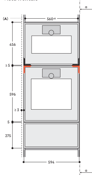
Vista frontale
