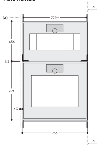
Vista frontale
