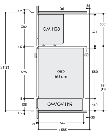
Vista laterale
