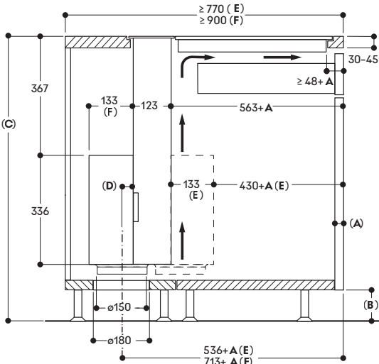
Vista laterale
