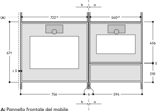
A: Pannello frontale del mobile
