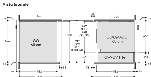
Vista laterale
