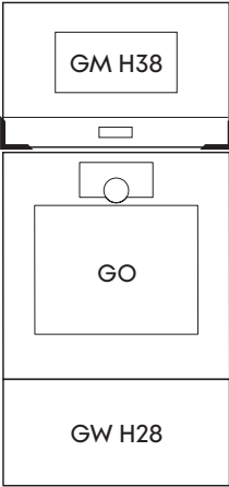
Combinazione MV6_28_H38 (Dimensioni, vedi pagina 68)
