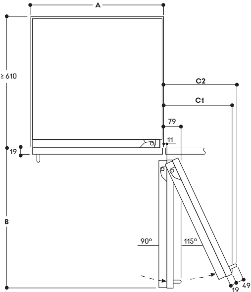
Larghezza della nicchia
