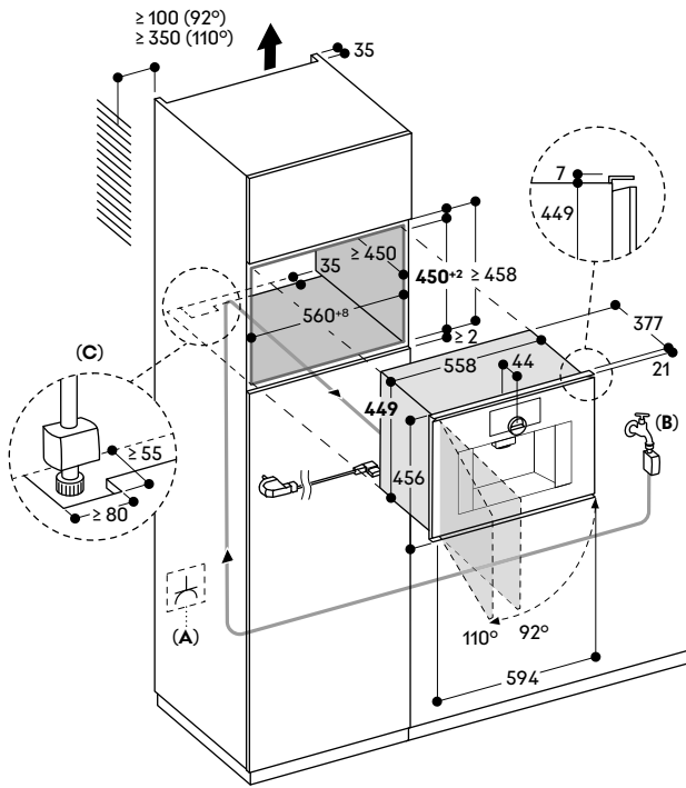
A: Presa elettrica B: Connessione alla rete idrica C: Taglio aggiuntivo per il passaggio dell'Aquastop
