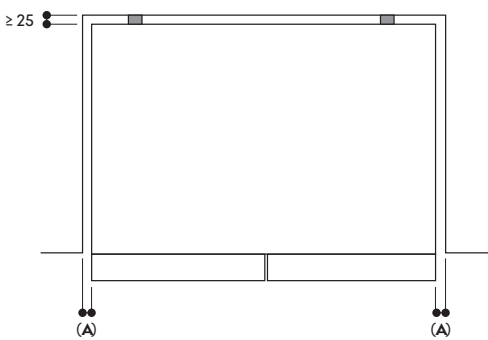
Distanze minime di installazione da pareti laterali
