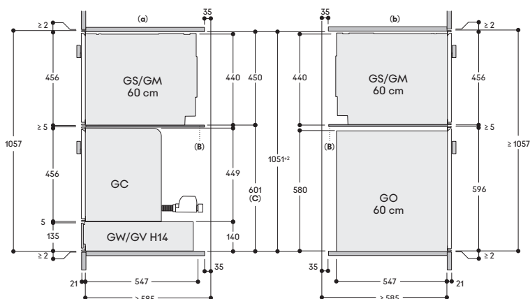
Vista laterale
