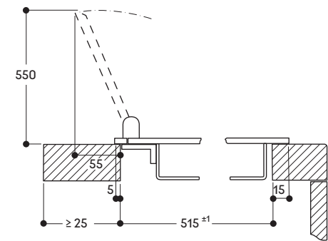
Installazione in appoggio con coperchio
