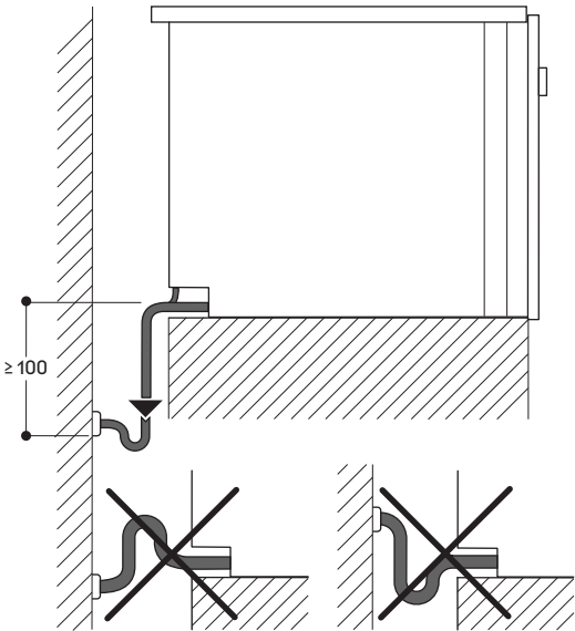
Vista da dietro
