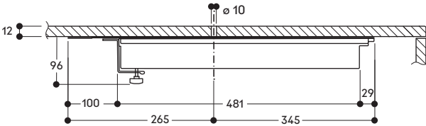
Sezione longitudinale
