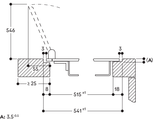
Installazione a filo con coperchio
