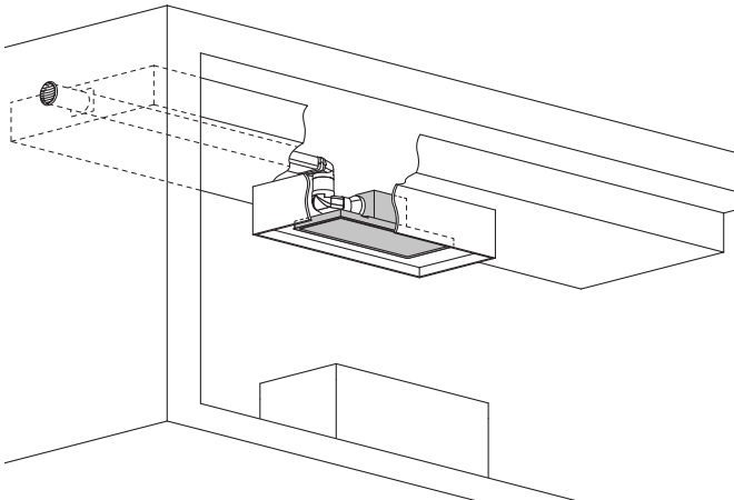
AC250 con collettore dei fumi Estrazione attraverso il controsoffitto
