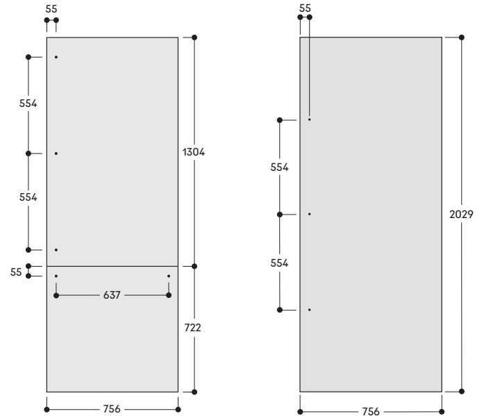
Apparecchi con larghezza nicchia 762 mm
