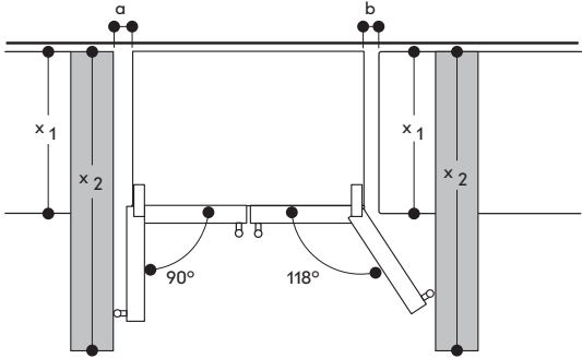
Angolo di apertura delle porte
