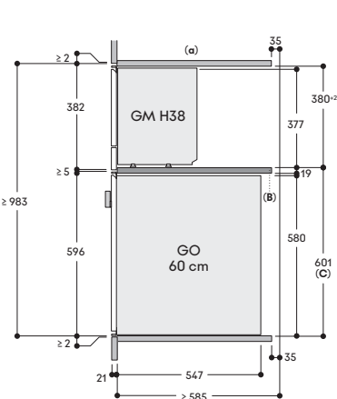
Vista laterale
