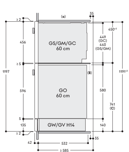
Vista laterale
