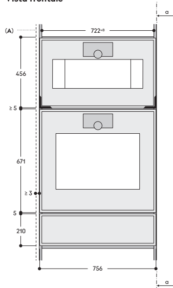
Vista frontale
