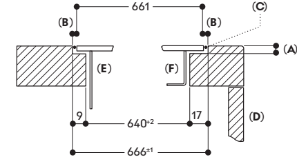
Sezione trasversale
