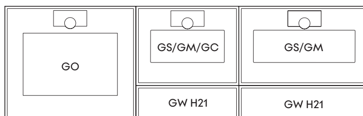
Combinazione EH363_21 (Dimensioni, vedi pagina 19)
