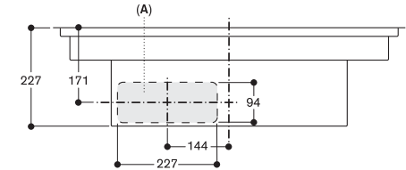
A: Connessione diretta dal retro
