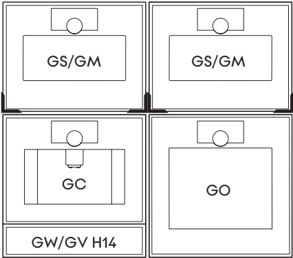
Combinazione ECU66_14_H45 (Dimensioni, vedi pagina 23)
