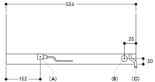
A: Morsettiera elettrica B: Scarico acqua C: Carico acqua fredda
