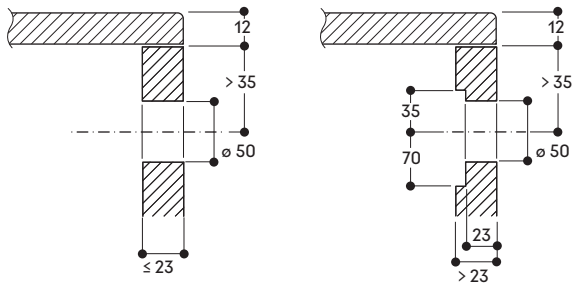
Installazione manopola
