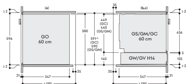
Vista laterale
