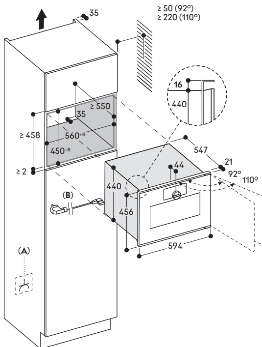
A: Presa elettrica B: Cavo con presa elettrica
