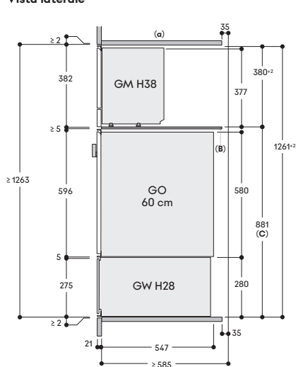
Vista laterale
