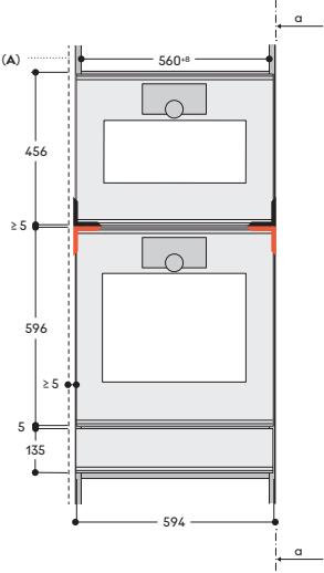
Vista frontale
