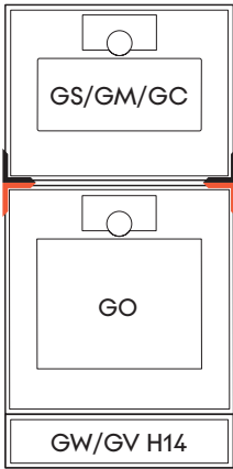
Combinazione EV6_14_H45 (Dimensioni, vedi pagina 20)
