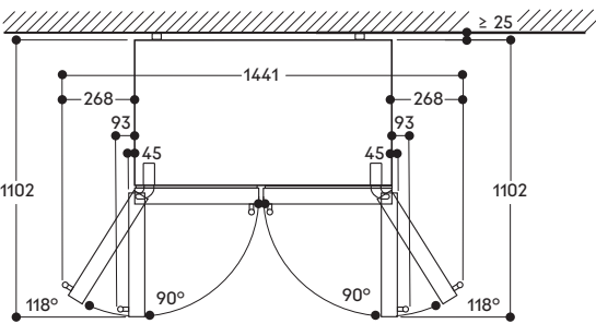
Distanze per l'apertura delle porte
