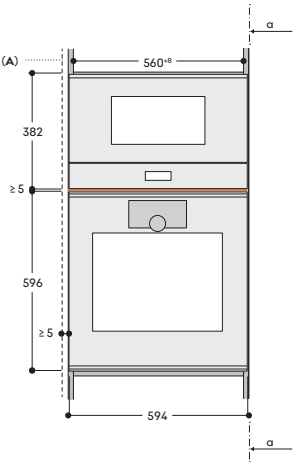
Vista frontale
