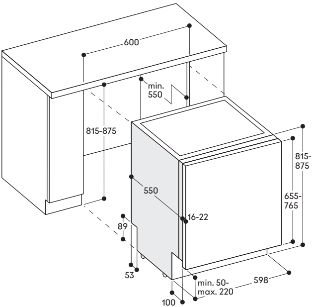
Altezza lavastoviglie 81,5 cm con cerniera sliding
