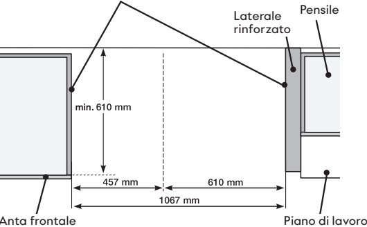
Nicchia. Taglio orizzontale
