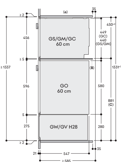
Vista laterale
