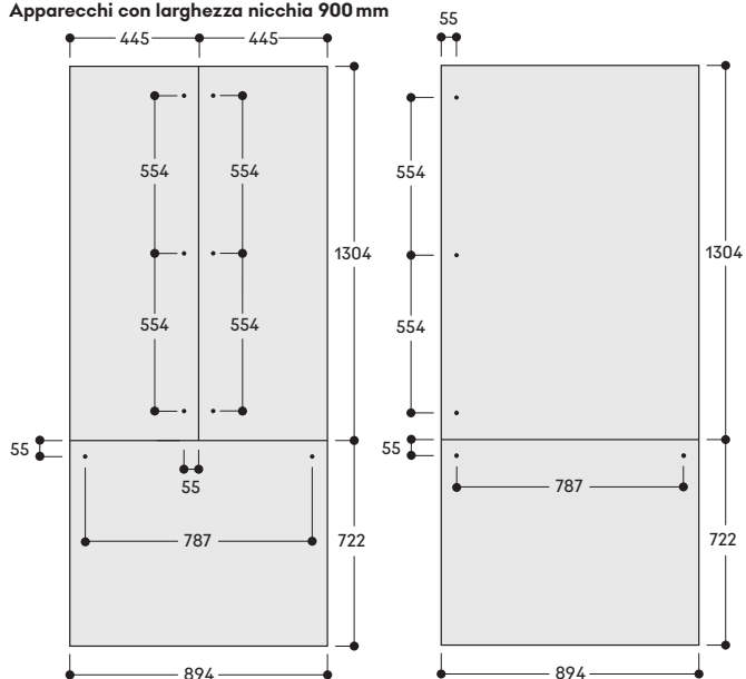
Apparecchi con larghezza nicchia 900 mm
