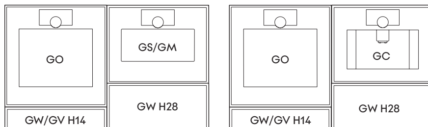
Combinazione EH66_1428 (Dimensioni, vedi pagina 18)
