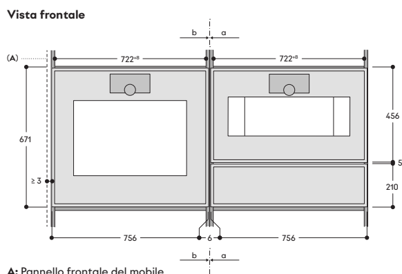
A: Pannello frontale del mobile
