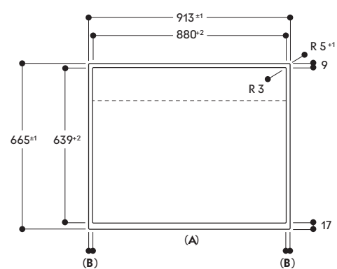
Vista dall'alto
