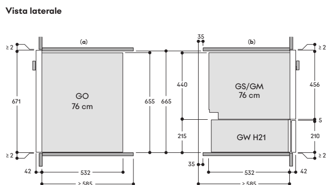
Vista laterale
