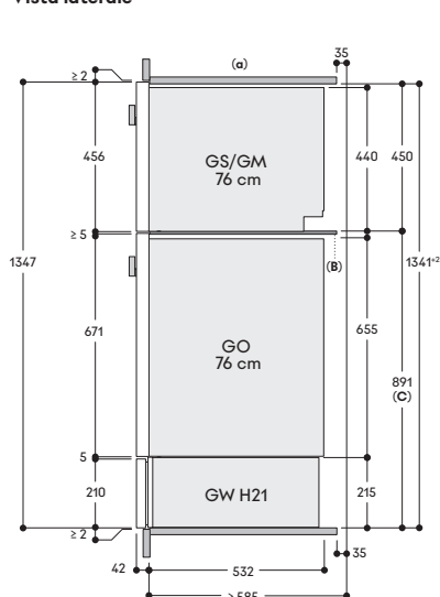
Vista laterale
