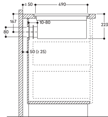
A: Per installazioni che prevedono il ricircolo dell'aria verso pareti posteriori non sufficientemente isolate (Trasmittanza termica U \geq 0.5 \text{ W/m}^2\text{K} ) si raccomanda una progettazione di tipo canalizzato.
