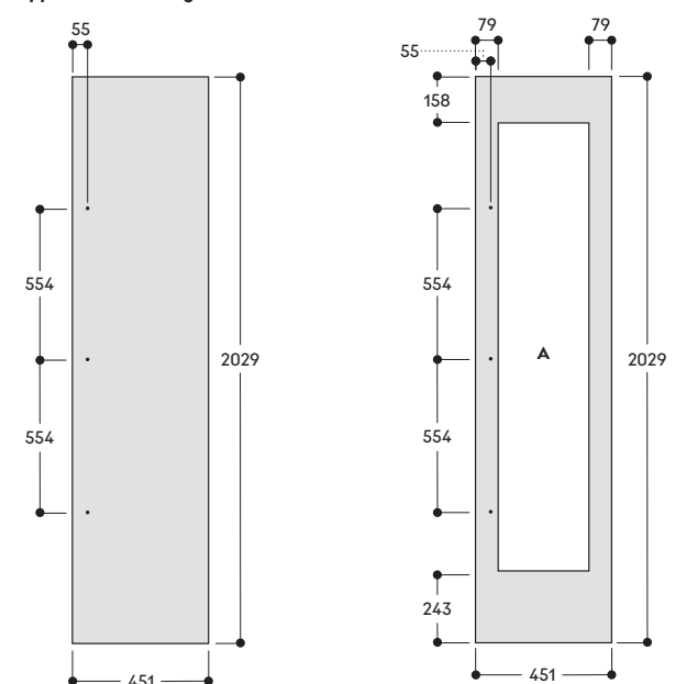
Apparecchi con larghezza nicchia 457 mm
