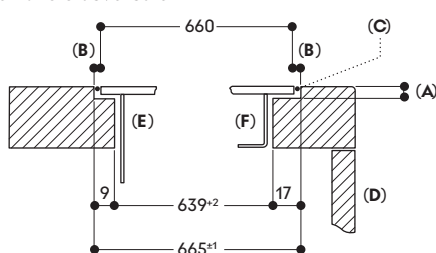
Sezione trasversale
