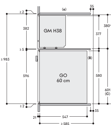
Vista laterale
