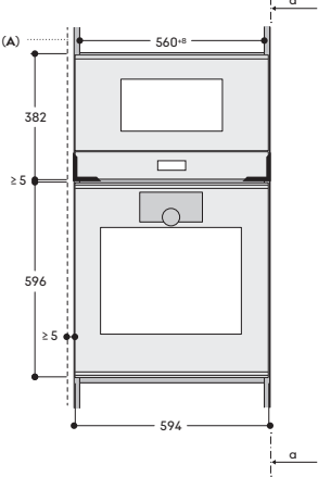
Vista frontale
