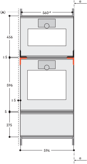
Vista frontale
