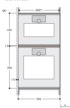
Vista frontale
