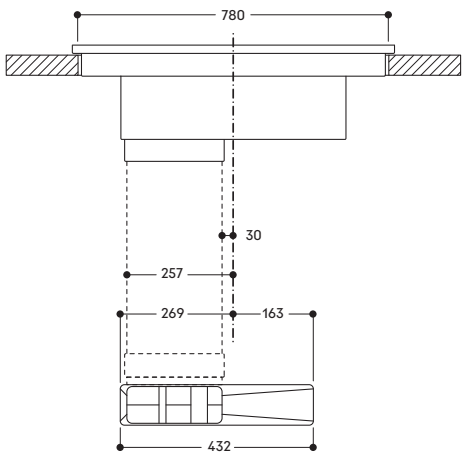
Vista frontale con ricircolo canalizzato
