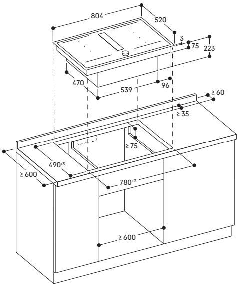
Installazione in appoggio
