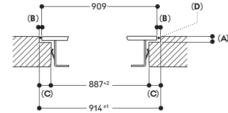
Sezione longitudinale
