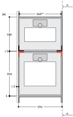
Vista frontale
