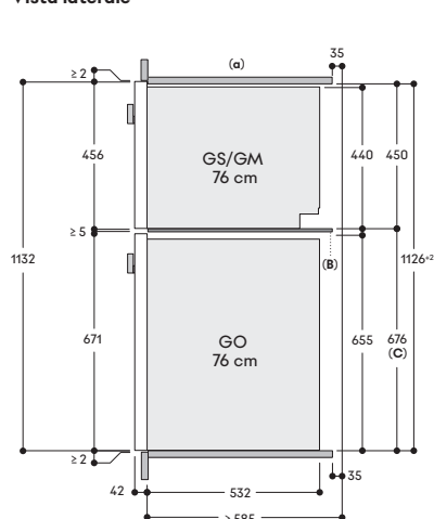
Vista laterale
