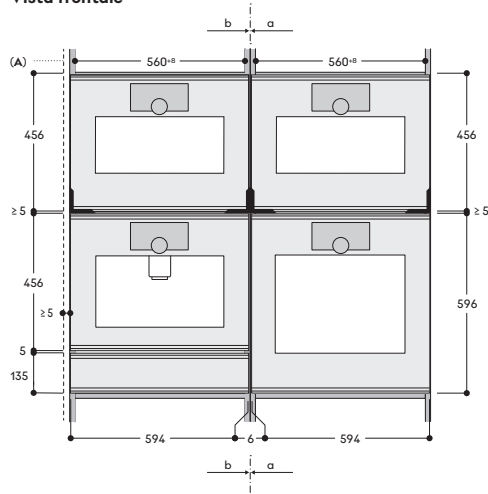
A: Frontale del mobile B: Ripiano intermedio C: Linea di riferimento
