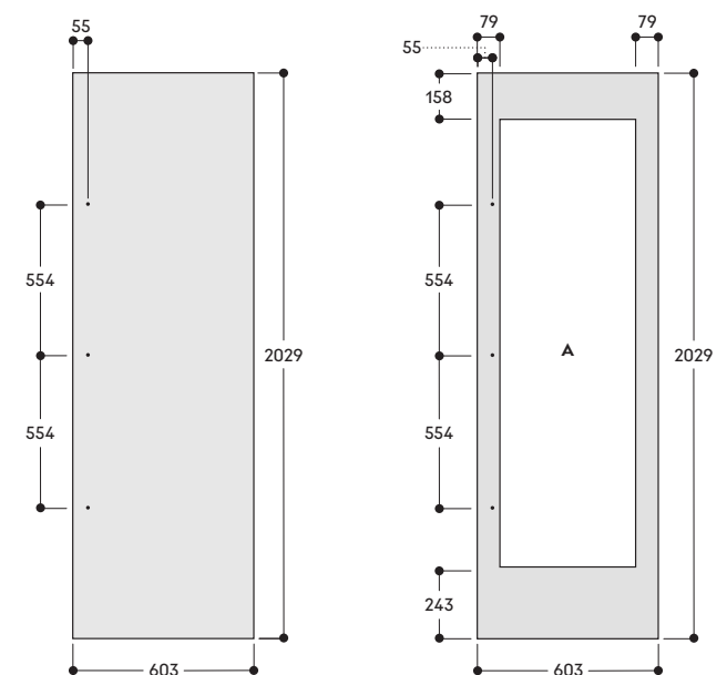
Apparecchi con larghezza nicchia 610 mm
