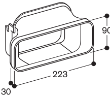
AD 851 041: Parte di connessione per estensione con tubo piatto DN 150 per piani di lavoro molto profondi
