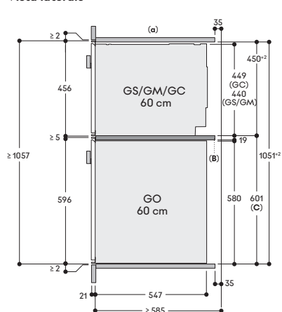
Vista laterale
