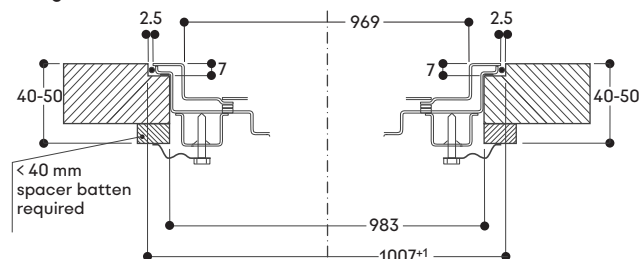
Longitudinal section
