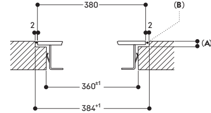
Longitudinal section
