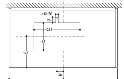
A: Cable bushing
