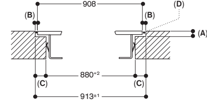
Longitudinal section
