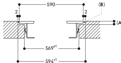
Longitudinal section
