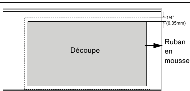
Figure 5: Découpe du comptoir – Pose d'un ruban en mousse
