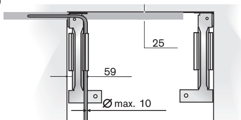
Plantegning
