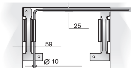
Vy ovanifrån
