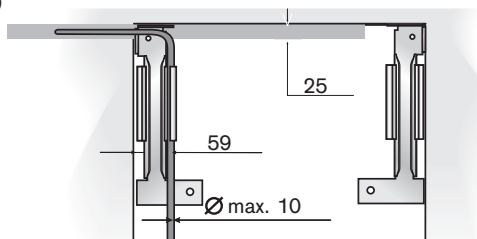
Vy ovanifrån
