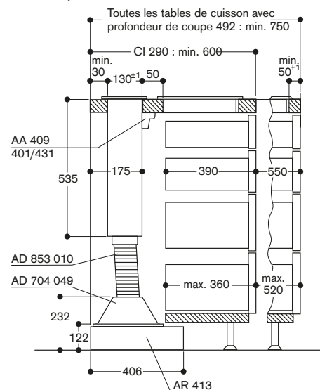
Section transversale du meuble bas pour AL 400 (sans paroi arrière) avec AR 413; raccordement vers le bas
