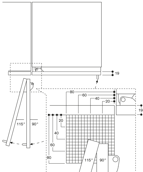
La course de la charnière et les distances en résultant par rapport au meuble avoisinant et aux poignées du meuble sont indiquées sur le schéma en fonction de l'épaisseur de la partie frontale. Sur ce schéma, l'épaisseur de la partie frontale utilisée est de 19 mm.
