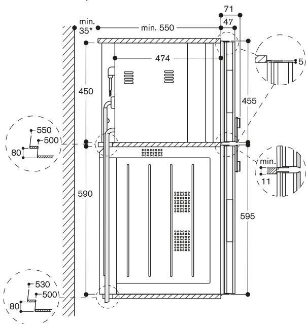
Vue latérale de BS 474/475 au-dessus de BO
