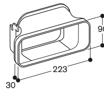
AD 851-041 : Pièce de connexion VL 200 pour extension avec conduit plat DN 150 pour un plan de travail très profond
