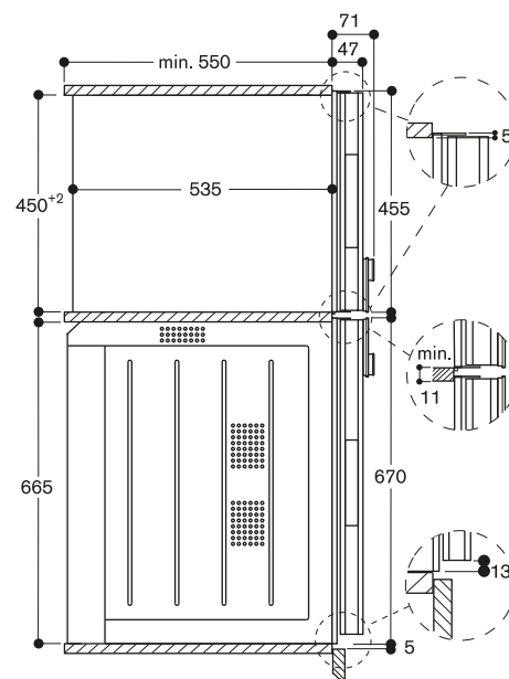
Vue latérale de BM 484/485 au-dessus de BO
