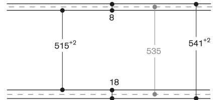
Avec recouvrement/baguette intercalaire
