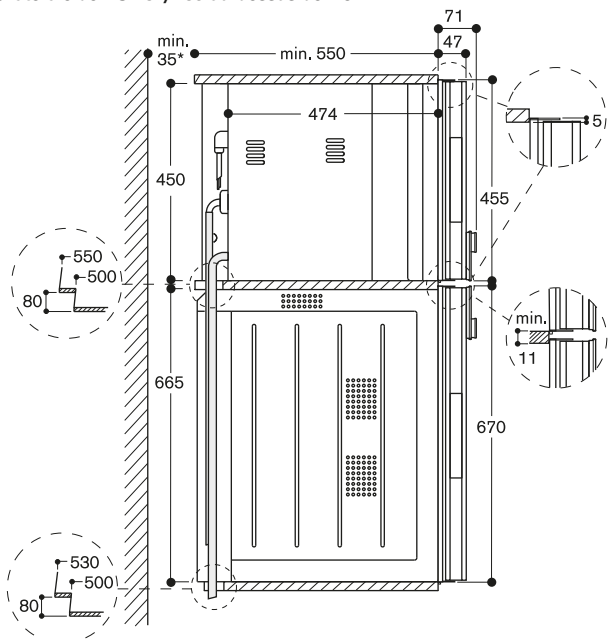
Vue latérale de BS 484/485 au-dessus de BO
