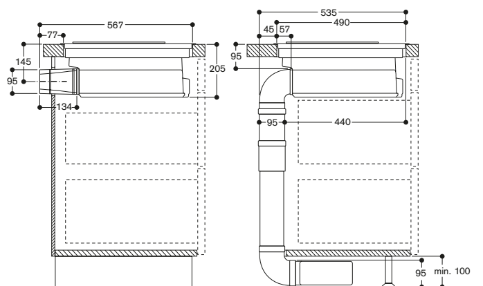
Vue de côté CV 282 avec pièce de connexion de la gaine plate CA 284-010
