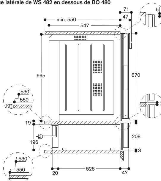
Vue latérale de WS 482 en dessous de BO 480
