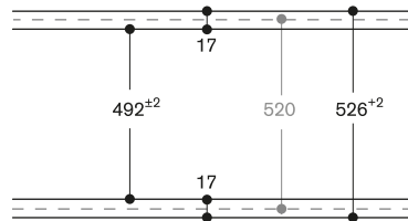
Sans recouvrement
