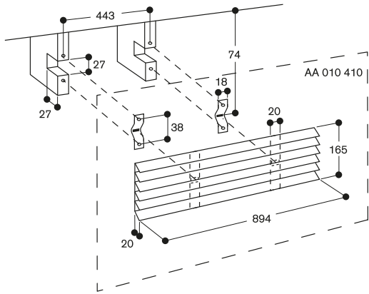
AA 010 410 Grille d'évacuation
