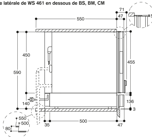
Vue latérale de WS 461 en dessous de BS, BM, CM
