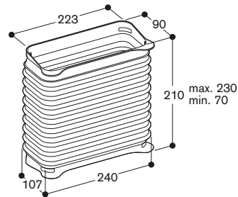
AD 410-040 : Pièce de connexion flexible pour VL 200, DN 150 plat
