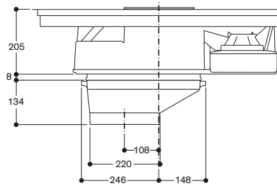
Vue de face CV 282 avec pièce de connexion de la gaine plate CA 284-010
