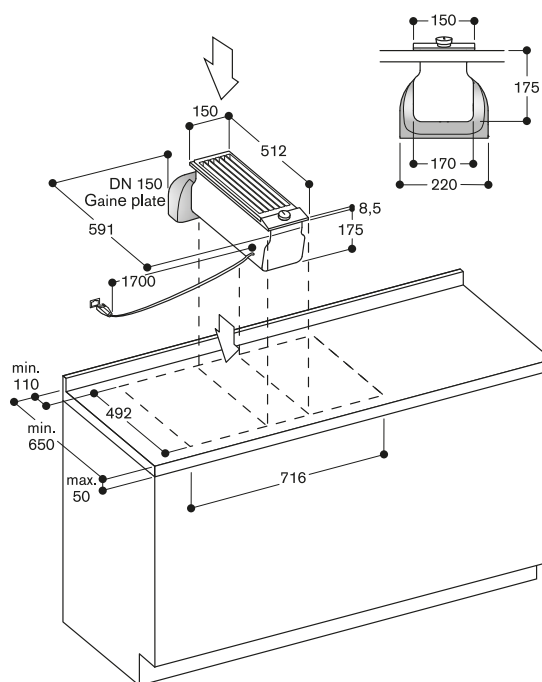
AD 410-040: pièce de connexion flexible pour VL 200, DN 150 plat.
