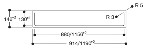
AL 400 découpe installation à fleur de plan
