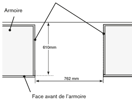
Vue de dessus de la niche d'installation
