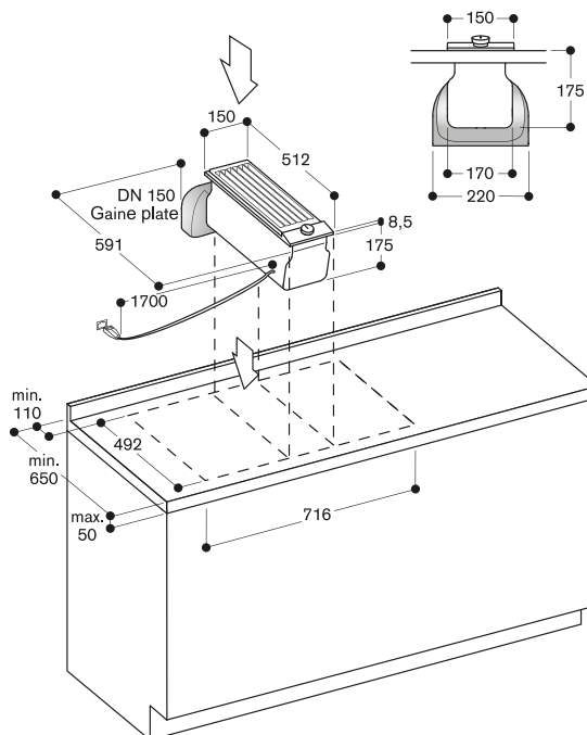
AD 410-040: pièce de connexion flexible pour VL 200, DN 150 plat.
