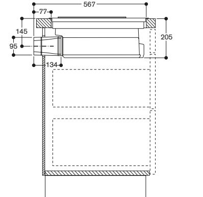
Vue de côté CV 282 avec pièce de connexion de la gaine plate CA 284-010
