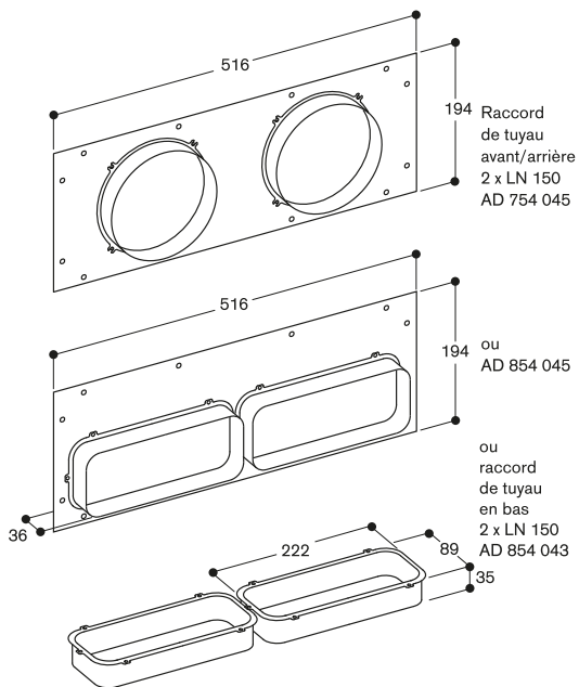
AD 754/854 045 et AD 854 043
