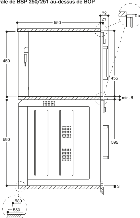
Vue latérale de BSP 250/251 au-dessus de BOP
