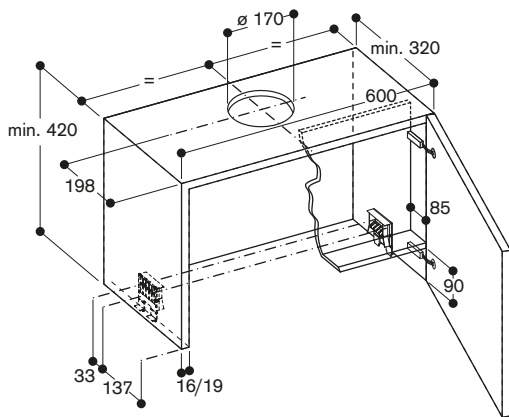
Meuble haut pour AF 200-160 avec kit de suspension hotte tiroir AA 210-460
