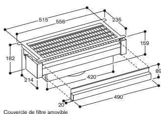
Couvercle de filtre amovible
