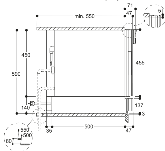
Vue latérale de DV 461 en dessous de BS, BM, CM
