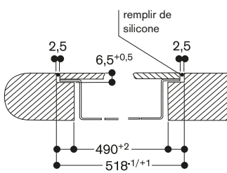
Coupe transversale
