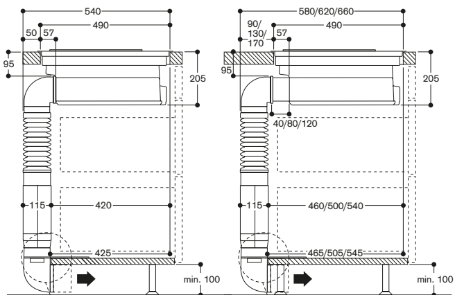
Vue de côté CV 282 avec module de recyclage de l'air CA 282-810
