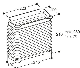
AD 410-040: pièce de connexion flexible pour VL 200, DN 150 plat.
