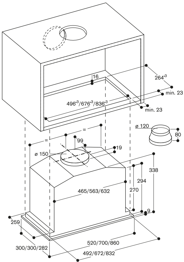
Vue du meuble haut du dessus avec AC 200 et AA 211-812
