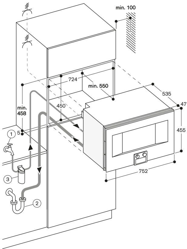
Vue latérale de BS 484/485 au-dessus de BO
