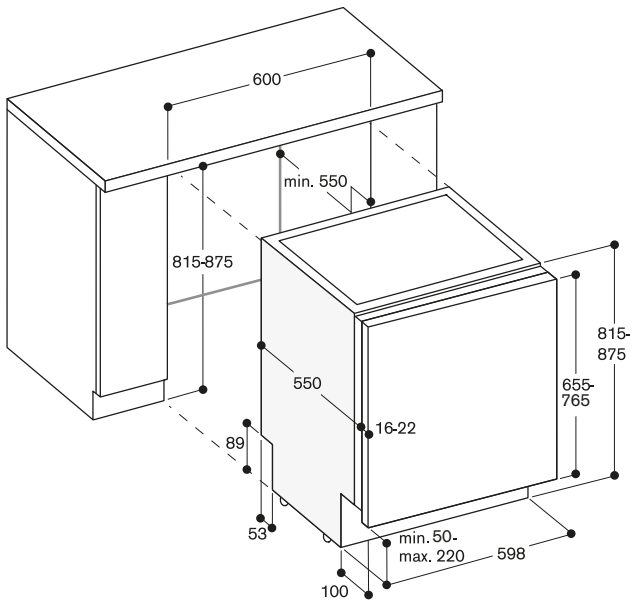
Lave-vaisselle 81,5 cm de haut avec charnières flexibles
