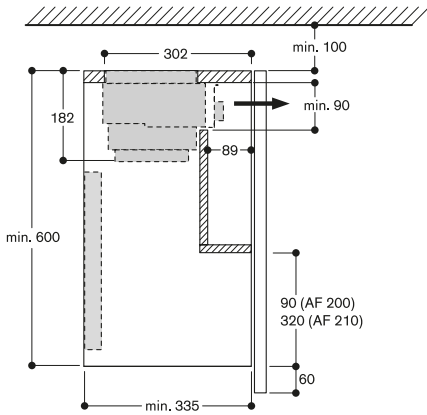
Section transversale du meuble haut avec AA 211-812 et kit de suspension hotte tiroir AA 210-490/460
