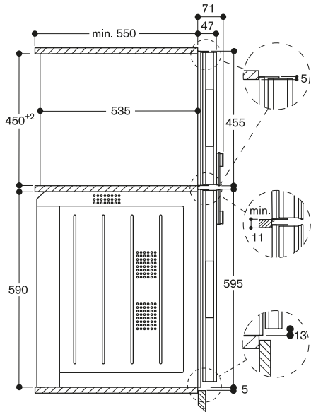
Vue latérale de BS454/455, BM 454/455 au-dessus de BO
