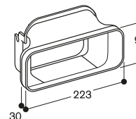
AD 851-041: pièce de connexion VL 200 pour extension avec conduit plat DN 150 lors d'un plan de travail très profond.
