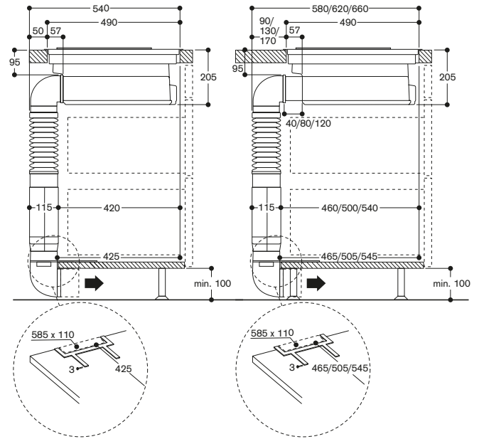
Vue de côté CV 282 avec module de recyclage de l'air CA 282-810
