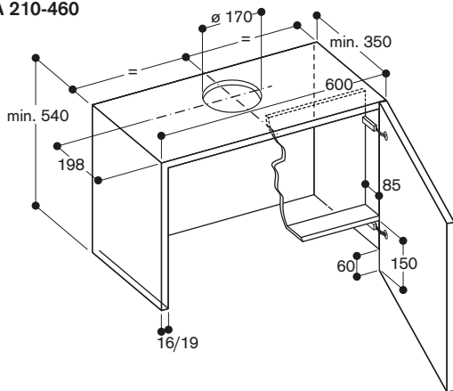
Section transversale du meuble haut avec AA 211-812 et kit de suspension hotte tiroir AA 210-490/460
