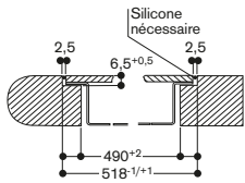
Coupe transversale
