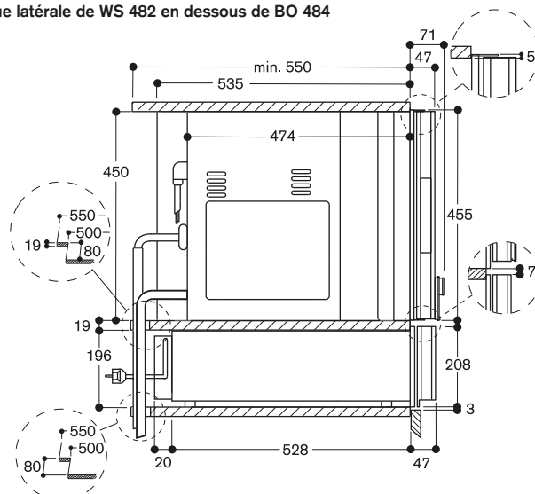
Vue latérale de WS 482 en dessous de BO 484
