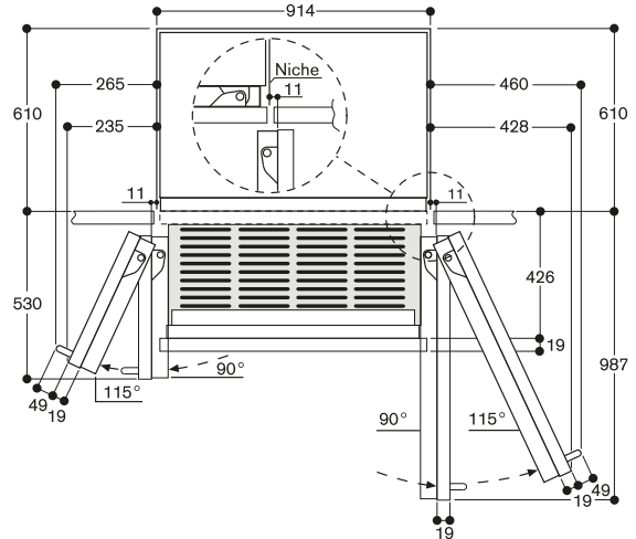
Le schéma suppose une épaisseur de partie frontale de 19 mm et une hauteur de 49 mm pour la poignée du meuble Gaggenau.
