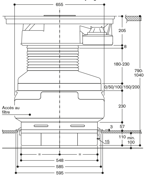
Vue de face CV 282 avec module de recyclage de l'air CA 282-810
