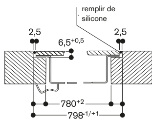
Coupe longitudinale
