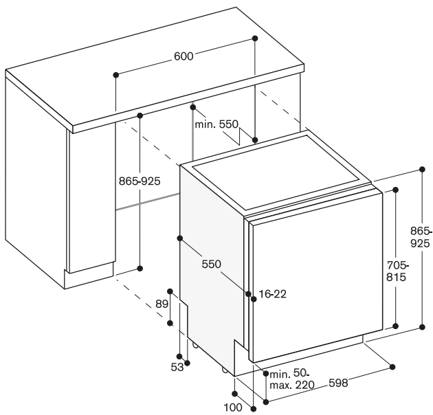
Lave-vaisselle 86,5 cm de haut avec charnières flexibles
