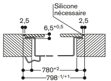
Coupe longitudinale
