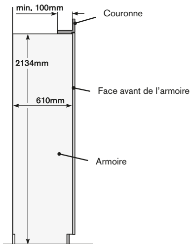
Vue de côté de la niche d'installation
