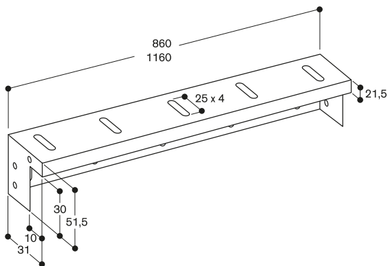
AA 409-401/431 traverse du meuble
