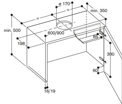
Meuble haut pour AF 210/211 avec kit de suspension hotte tiroir AA 210-460 / AA 210-490
