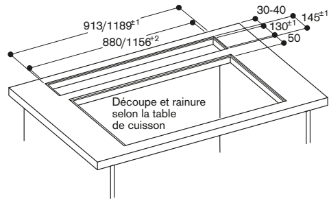
AL 400 installation à fleur de plan
