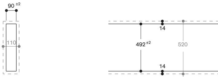
Sans recouvrement
