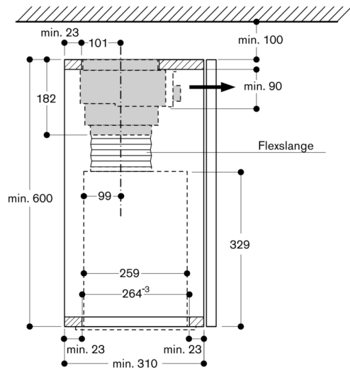
Tværsnit af overskab med AC 200 og AA 211 812
