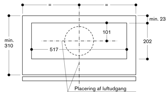
Overskab vist fra oven med AC 200 og AA 211 812
