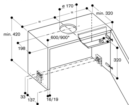
Overskab til AF 210
