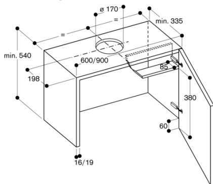
Overskab til AF 210 med nedsænkingsramme AA 210 460 / AA 210 490
