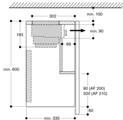
Tværsnit af overskab med AA 211 812 og nedsænkingsramme AA 210 490/460
