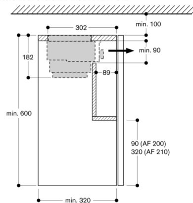
Tværsnit af overskab med AA 211 812
