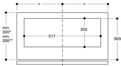
Overskab vist fra oven med AA 211 812
