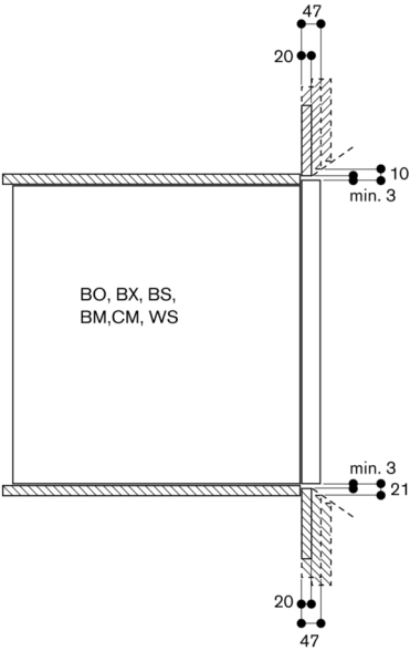
Areal af luftåbninger ved lågekanter oppe/nede
