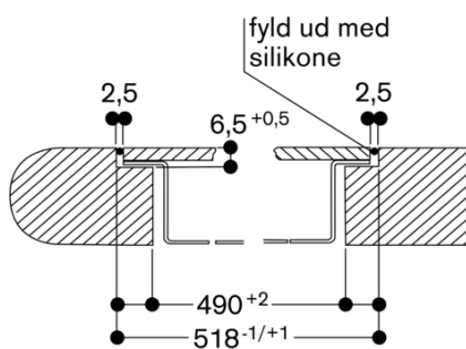
Tværsnit
