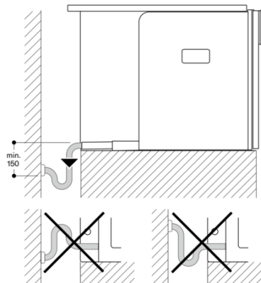
Afløbsvandstilslutning
