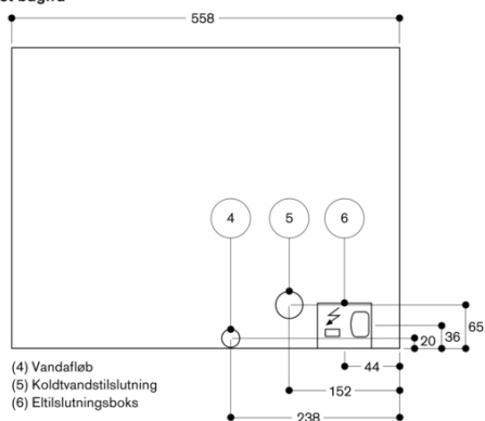
Set bagfra
