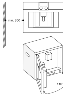
Hjørneindbygning venstre
