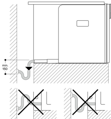
Afløbsvandtilslutning
