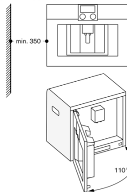
Hjørneindbygning venstre
