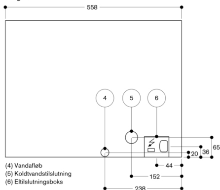
Set bagfra
