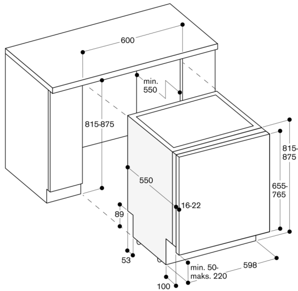
81,5 cm høj opvaskemaskine med fleksibelt hængsel
