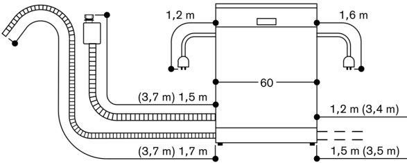
Tilslutningsmål for en 60 cm bred opvaskemaskine
