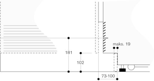
Detaljeudsnit - sokkel
