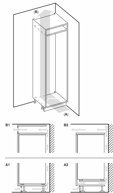
A: Luftindtag \geq 200 \text{ cm}^2 , ventilationsmuligheder A1 eller A2 B: Luftaftræk \geq 200 \text{ cm}^2 , ventilationsmuligheder B1 eller B2
