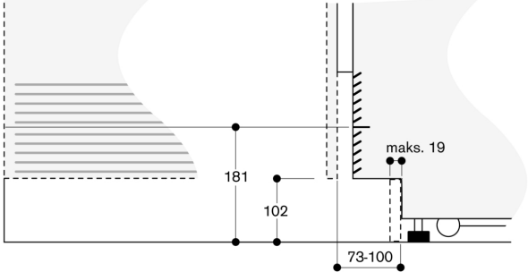
Detaljeudsnit - sokkel
