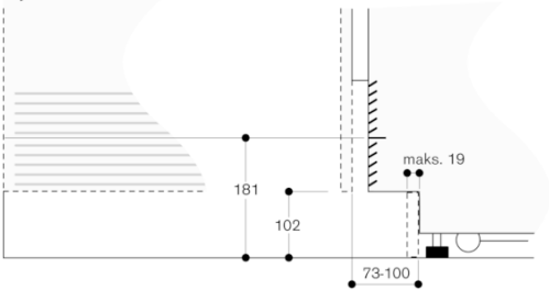
Detaljeudsnit - sokkel
