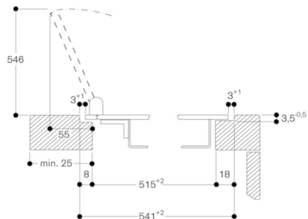
Installation med afdækning / udligningsliste, planforsænket montering
