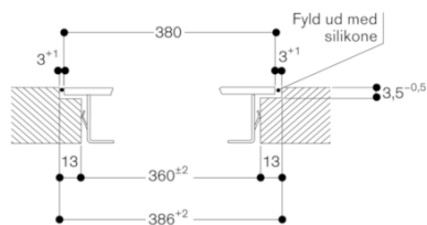
Længdesnit
