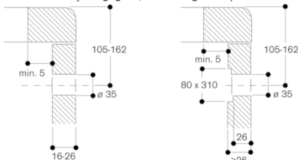
Installation af betjeningsgreb, montering oven på hinanden
