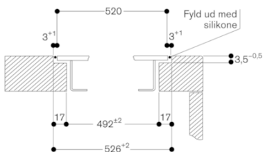
Tværsnit
