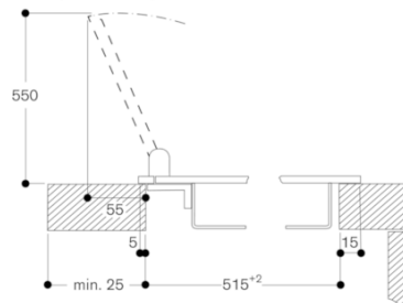
Installation med afdækning / udligningsliste, udvendig montering
