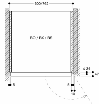
Luftquerschnitt an den Türkanten
