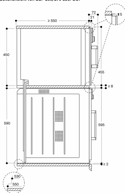
Seitenansicht von BSP 260/270 über BOP
