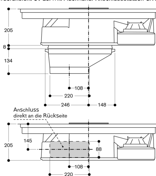
Vorderansicht CV 28. mit Flachkanal-Anschlussstutzen CA 284 011
