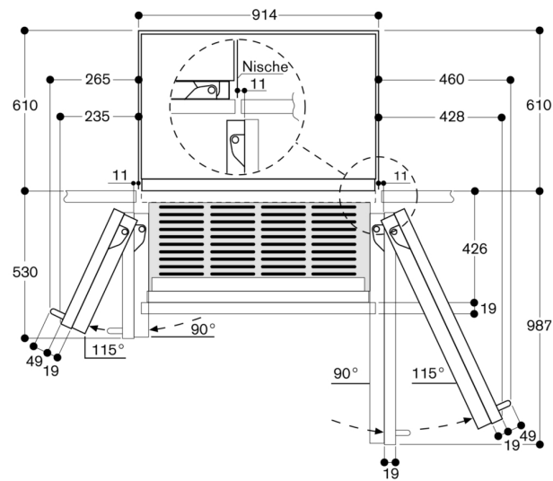
Wandabstand RB 492/RY 492
