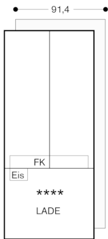
Wandabstand RB 492/RY 492
