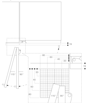
Türöffnungswinkel
