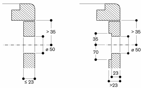
Montage Bedienknebel, flächenbündiger Einbau
