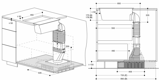
A: Aufbaumontage B: Flächenbündiger Einbau (nur VL 414) C: Filterzugang von der Vorderseite D: Filterzugang von der Rückseite Nicht empfohlen für nicht wärmeisolierte Böden ( U \geq 0,5 \text{ W/m}^2\text{K} ) Maße in mm
