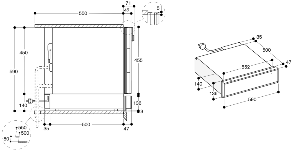
Seitenansicht WS 461 unter BS, BM, CM
