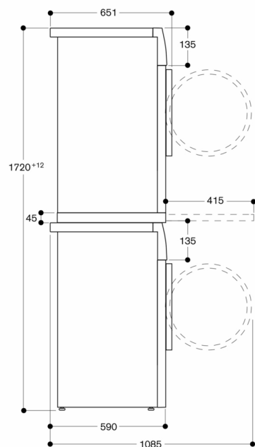
Seitenansicht von WT 260 über WM 260 mit Verbindungssatz-Zubehör
