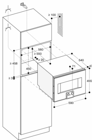
1 Steckdose Masse in mm
