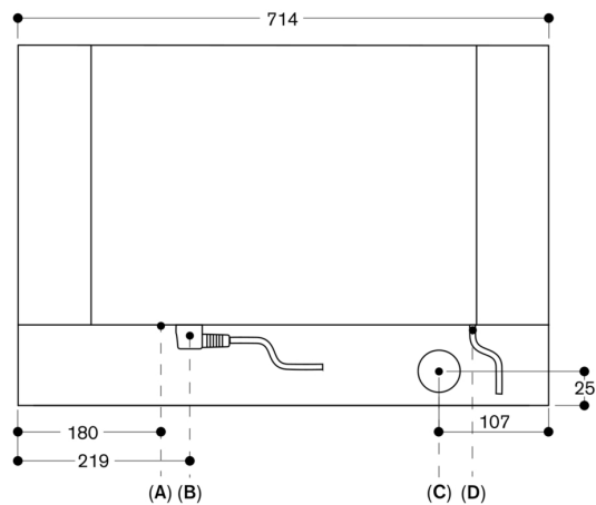
Ansicht von hinten
