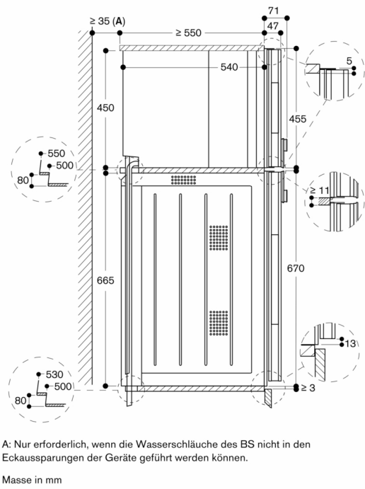
Seitenansicht BS 484/485 über BO
