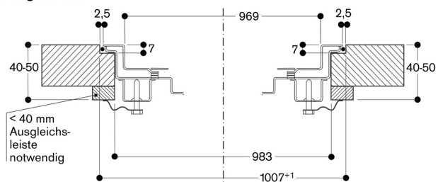
Längsschnitt
