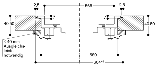
Querschnitt
