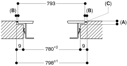
Längsschnitt
