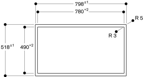
Ansicht von oben
