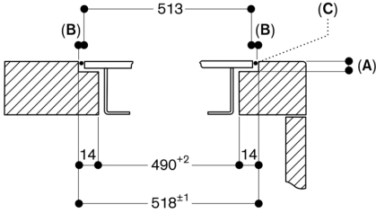
Querschnitt
