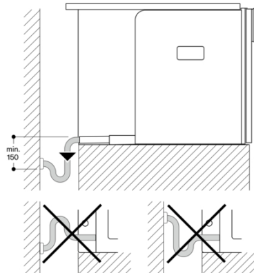
Abwasseranschluss
