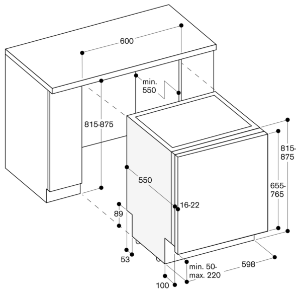
81,5 cm hoher Geschirrspüler mit flexiblem Scharnier
