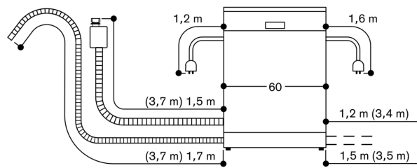
Anschlussmasse für einen 60 cm breiten Geschirrspüler
