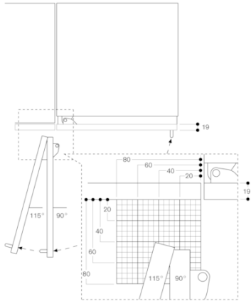
Türöffnungswinkel
