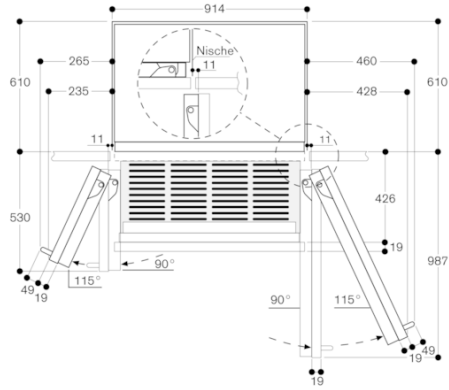
Wandabstand RB 492/RY 492
