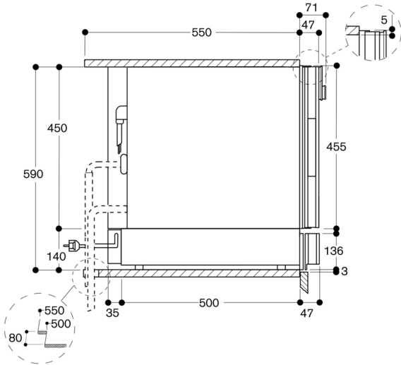
Seitenansicht WS 461 unter BS, BM, CM
