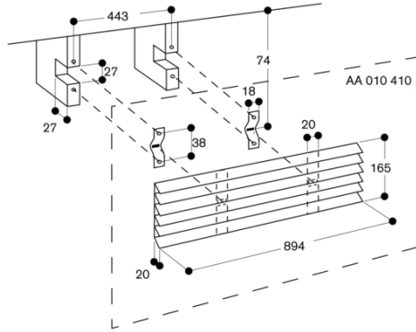
AA 010 410 Luftauslassgitter
