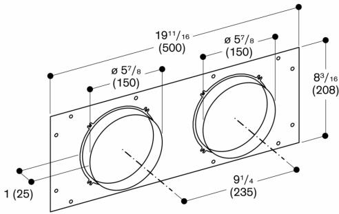
Maße in Zoll (mm)
