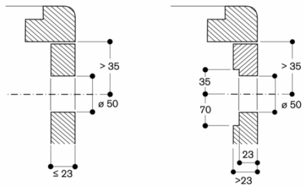
Montage Bedienknebel, flächenbündiger Einbau
