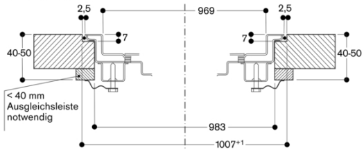
Längsschnitt
