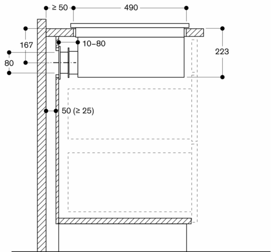
Seitenansicht mit ungeführter Umluft; aufgesetzt eingebaut
