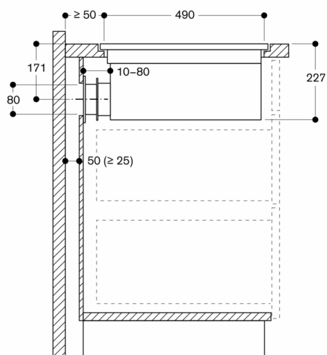
Seitenansicht mit ungeführter Umluft; flächenbündiger Einbau
