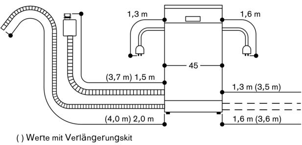
Anschlussmaße für einen 45 cm breiten Geschirrspüler
